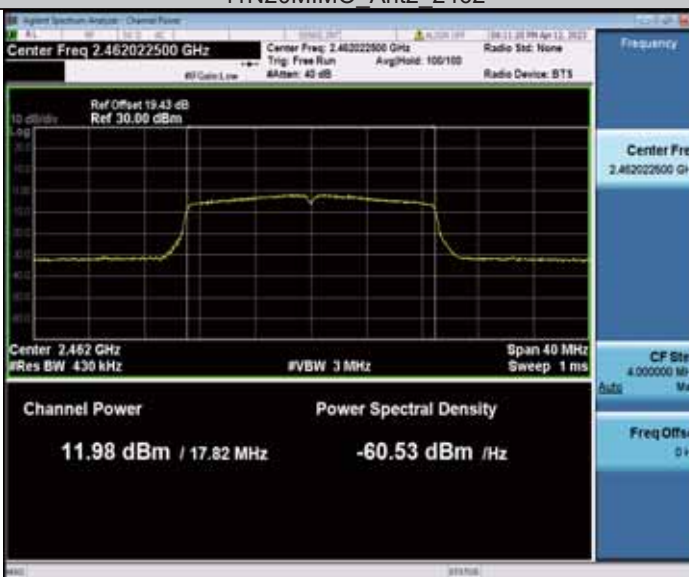
11N20MIMO_Ant2_2462
