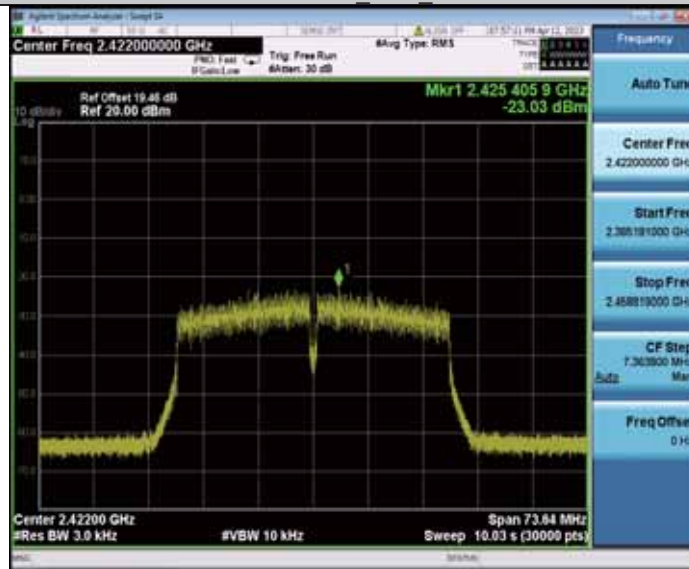
11N40MIMO_Ant2_242Z
