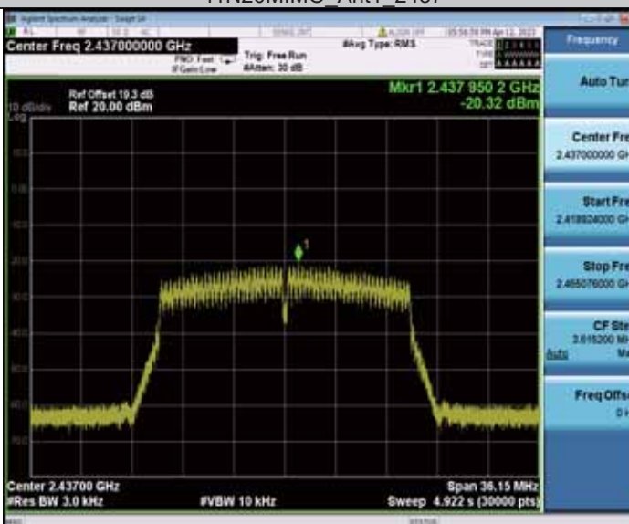
11N20MIMO_Ant1_2437
