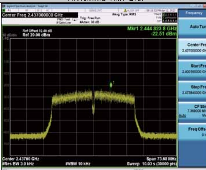
11N40MIMO_Ant1_243Z
