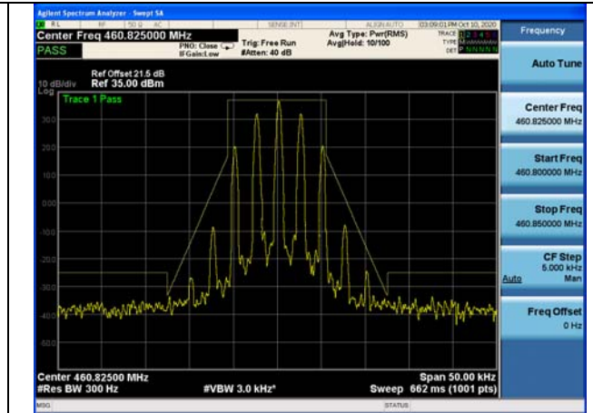
CH2
