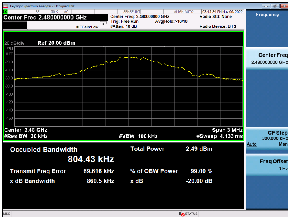
GFSK 2480MHz
