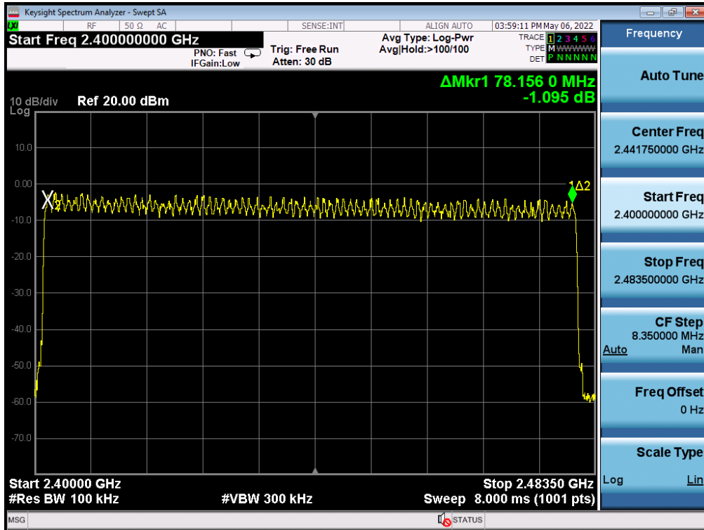
\pi/4 DQPSK
