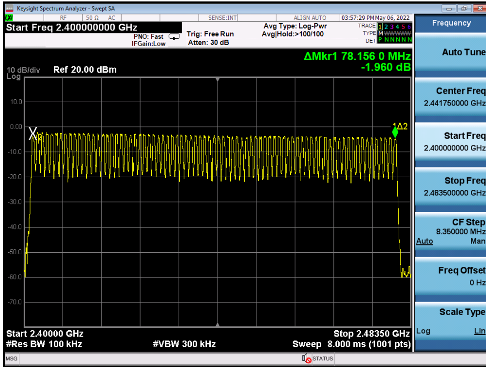
GFSK
