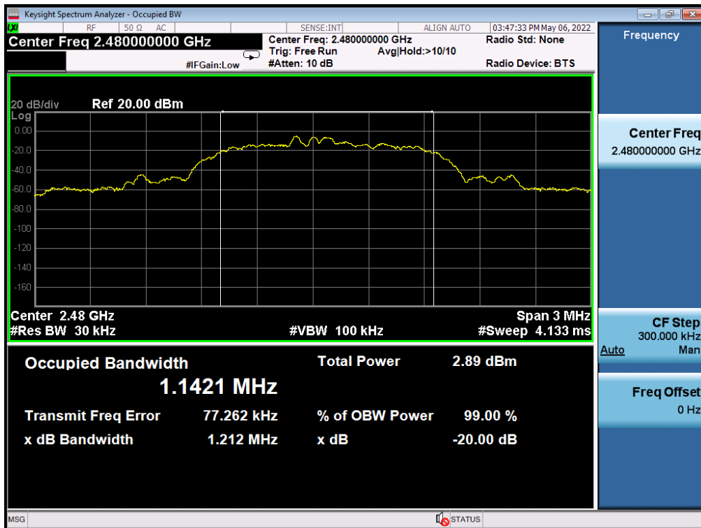
8DPSK 2480MHz
