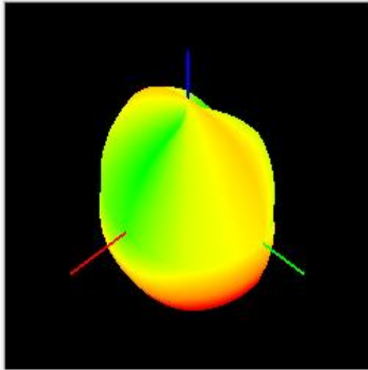
FDD-B5- TRP
