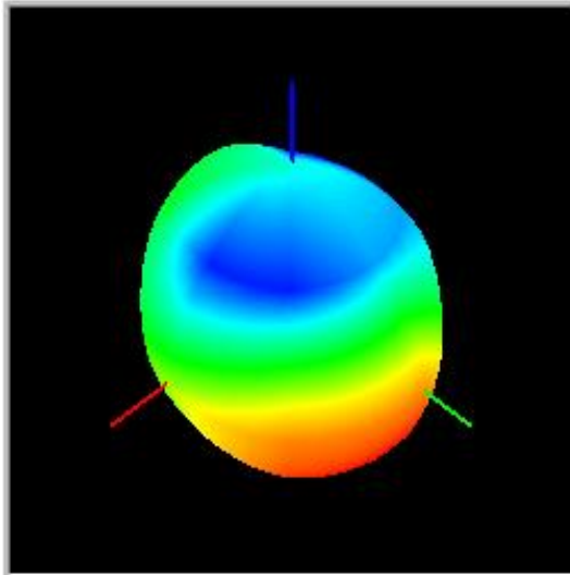
W4-TRP
