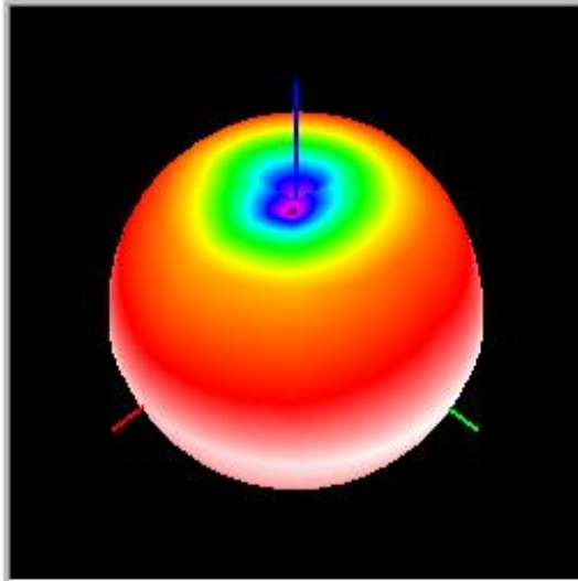
GSM850 -TRP
