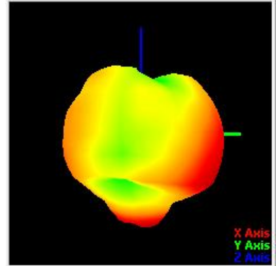
WIFI+BT- 2490MHZ
