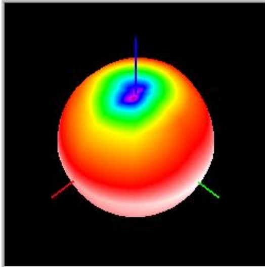
GSM900 -TRP
