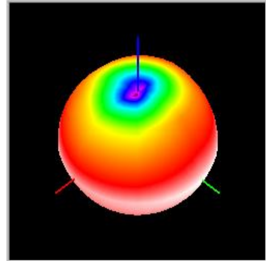
GSM850 -TIS
