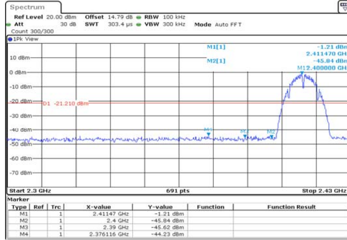
11B_Ant1_Low_2412
