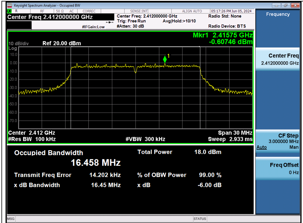
Test_Graph_802.11g_ANT1_2412_6Mbps_DTSSW
