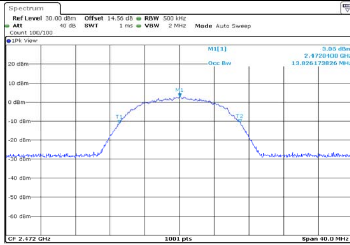
11B_Ant1_2472
