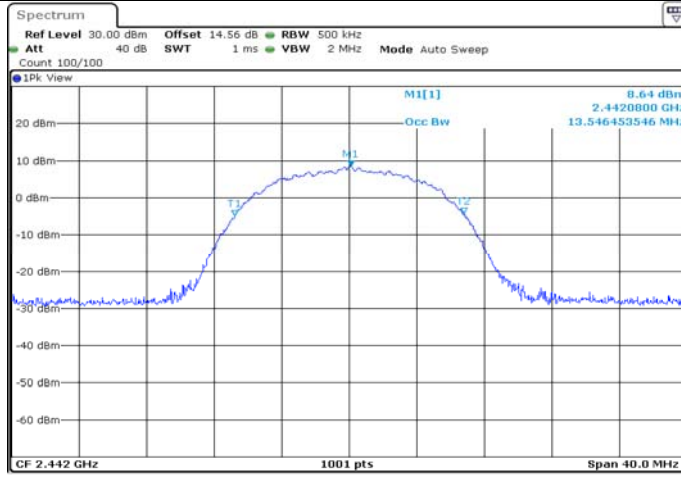
11B_Ant1_2442
