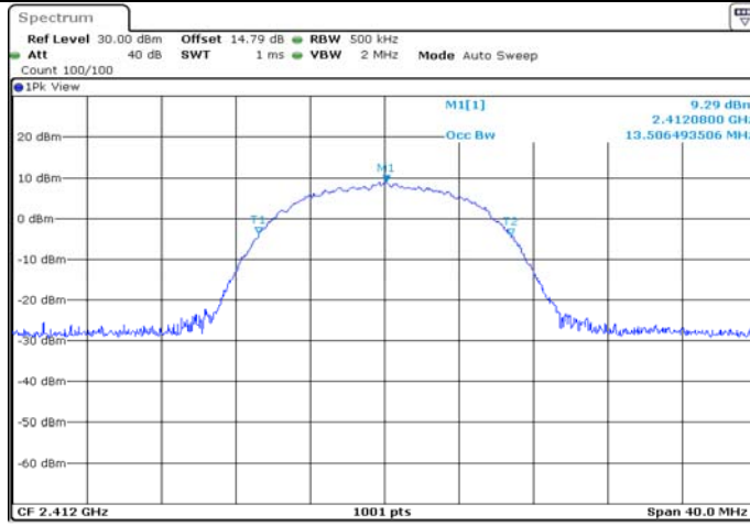
11B_Ant1_2412
