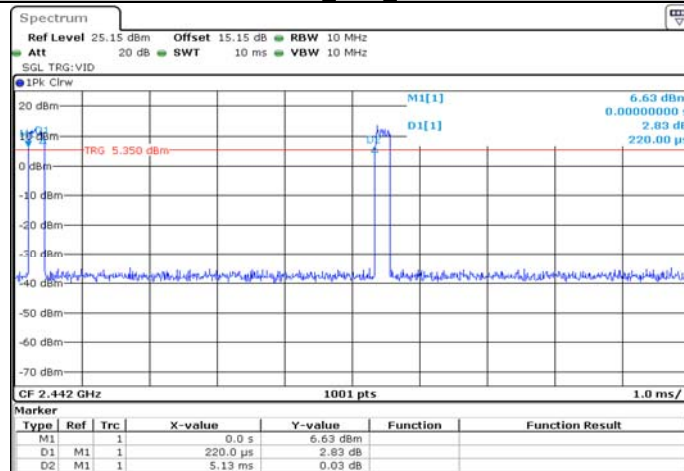
11N20_Ant1_2442
