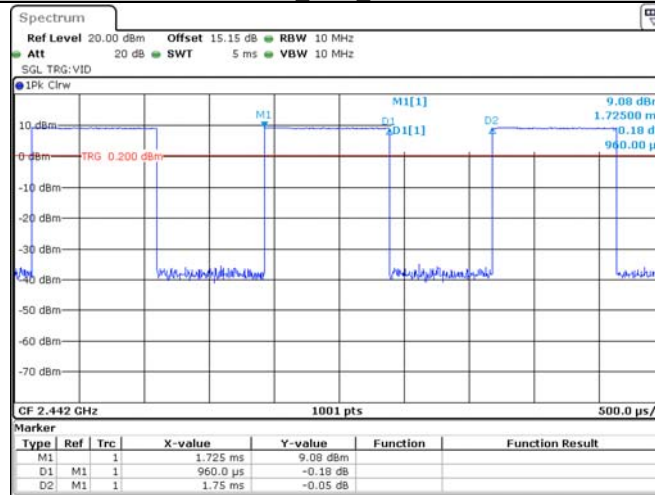
11B_Ant1_2442
