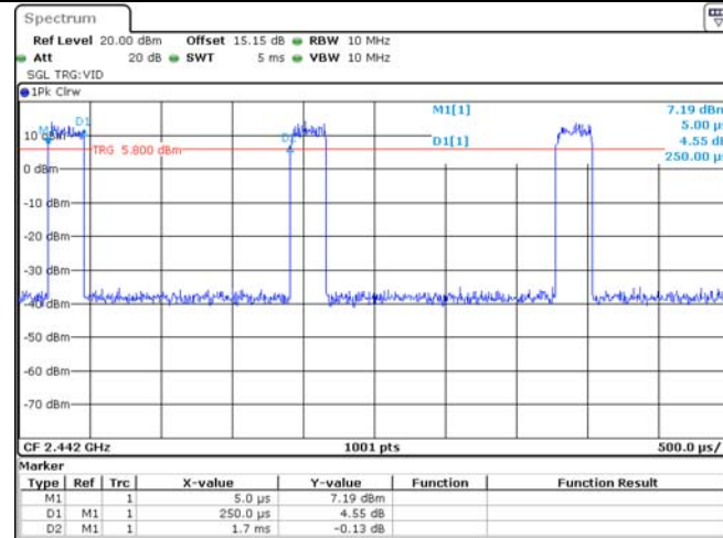
11G_Ant1_2442
