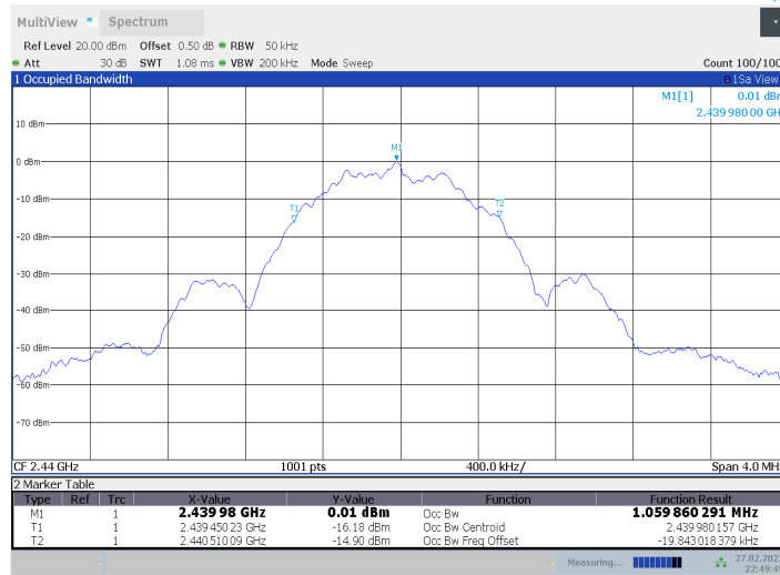
BLE_1M_Ant2_2440
