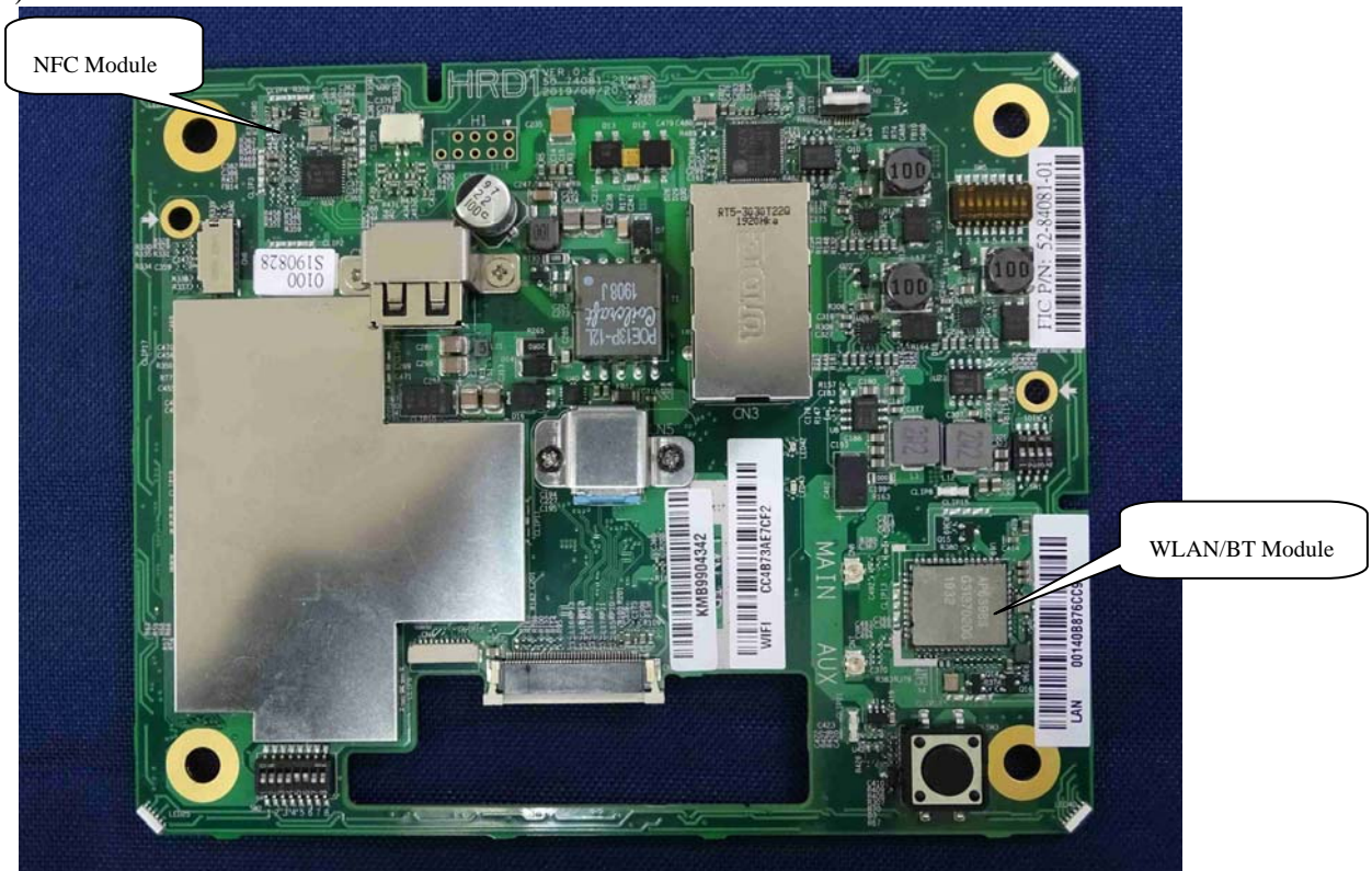
(16) EUT Photo
