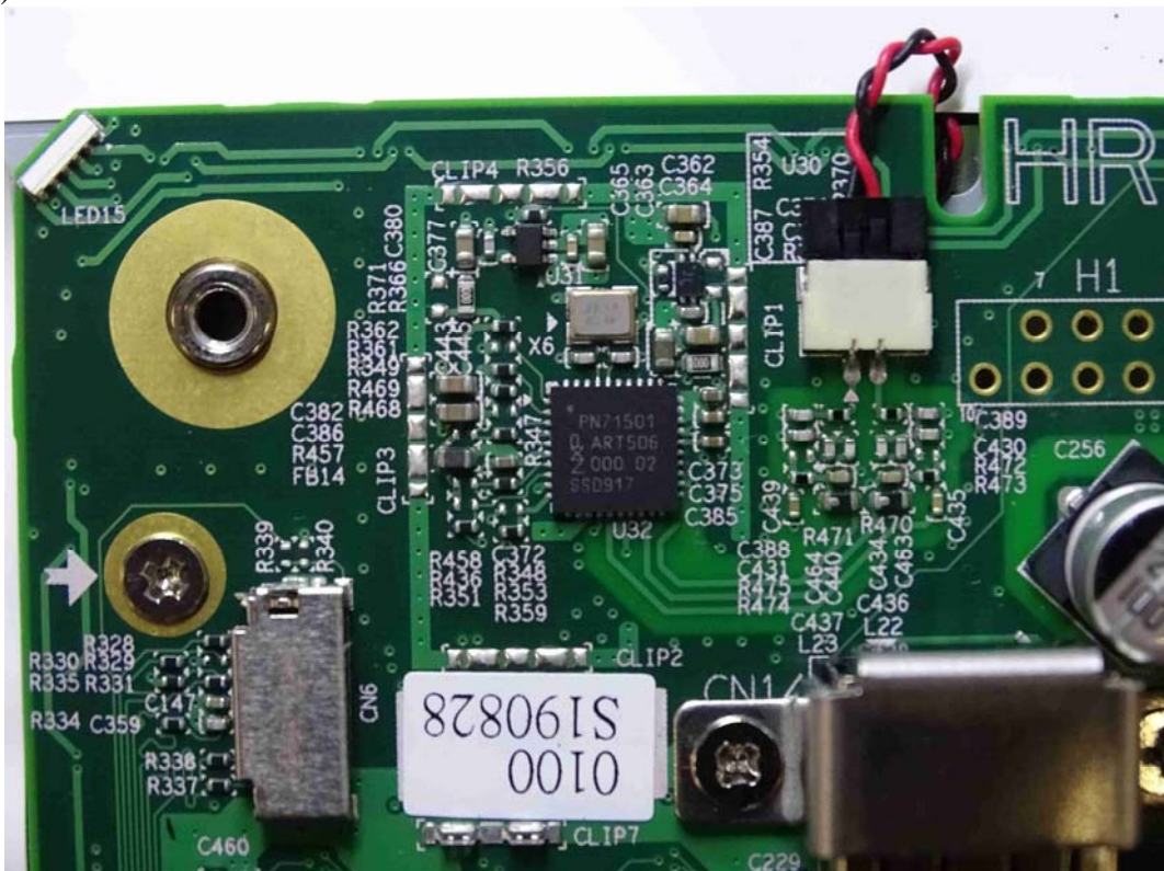
(20) EUT Photo-NFC Module
