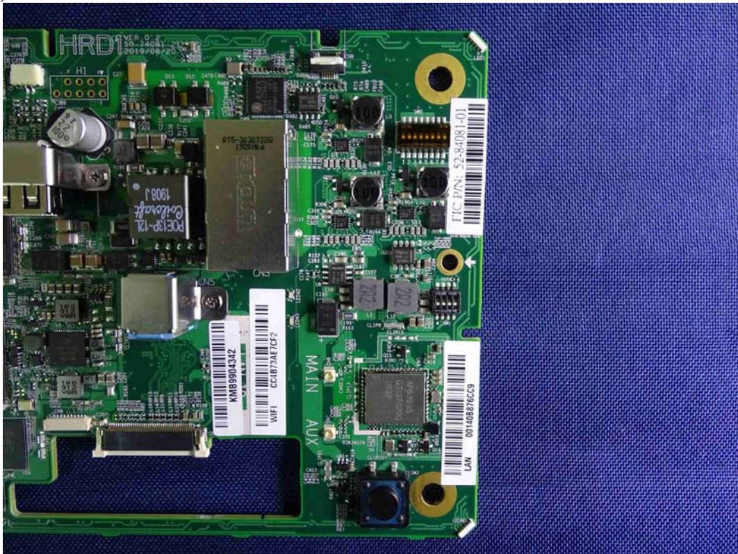
(22) EUT Photo-WLAN/BT Module
