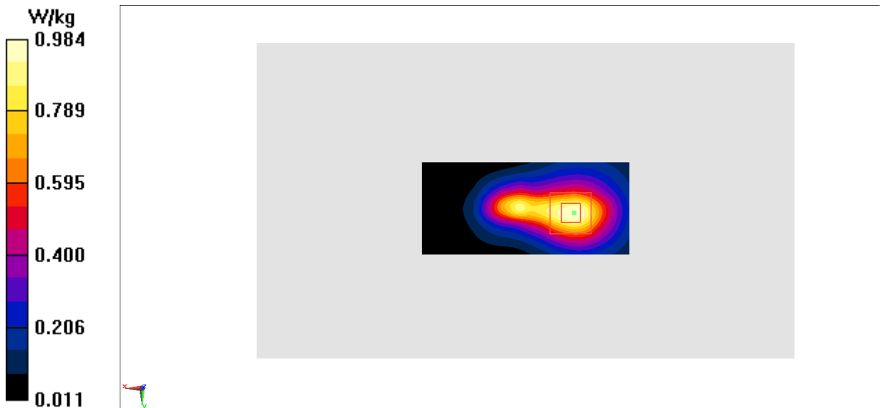
Fig.10 LTE Band7
