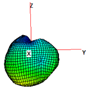
ant5 2410MHZ
