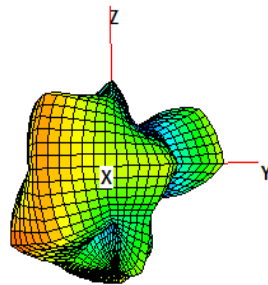
ant5 5500MHZ
