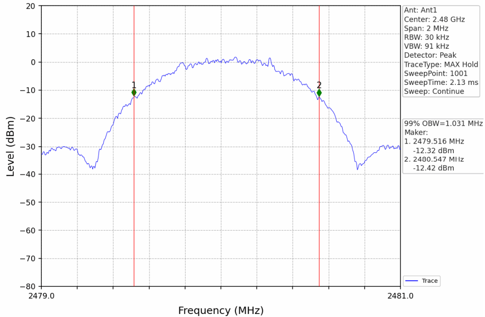
1M_HCH_2480MHz_DataRate=_Ant1_NTNV
