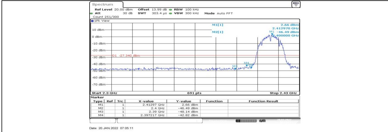
11B_Ant1_Low_2412
