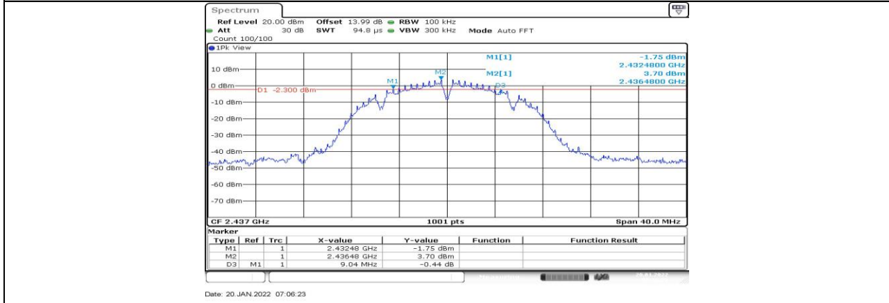
11B_Ant1_2437
