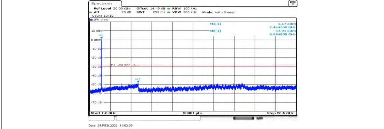
11G Ant1 2437 1000~26500
