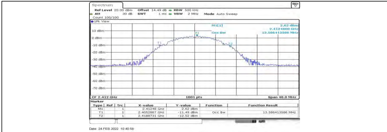
11B_Ant1_2412
