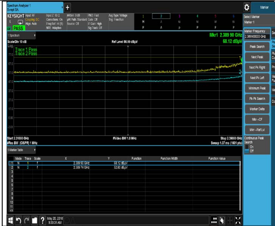
802.11n-HT20-2412MHz
