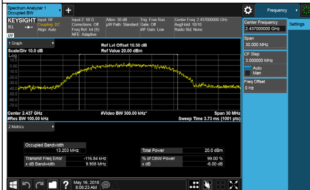
802.11b-2437MHz
