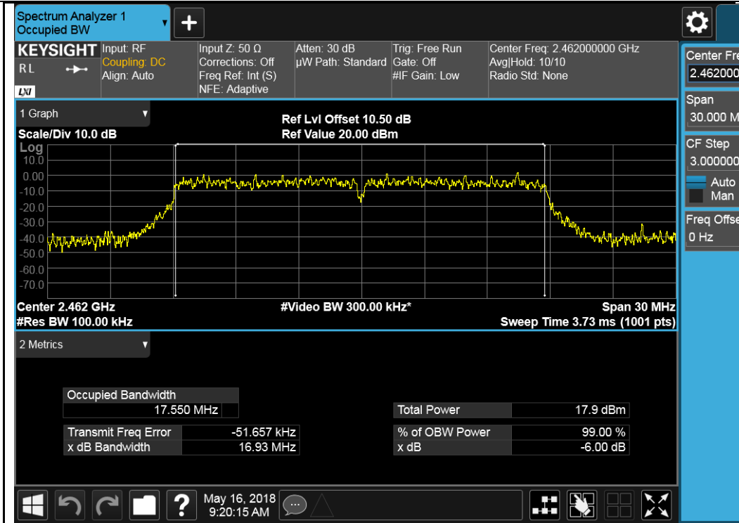
802.11n-HT20-2462MHz
