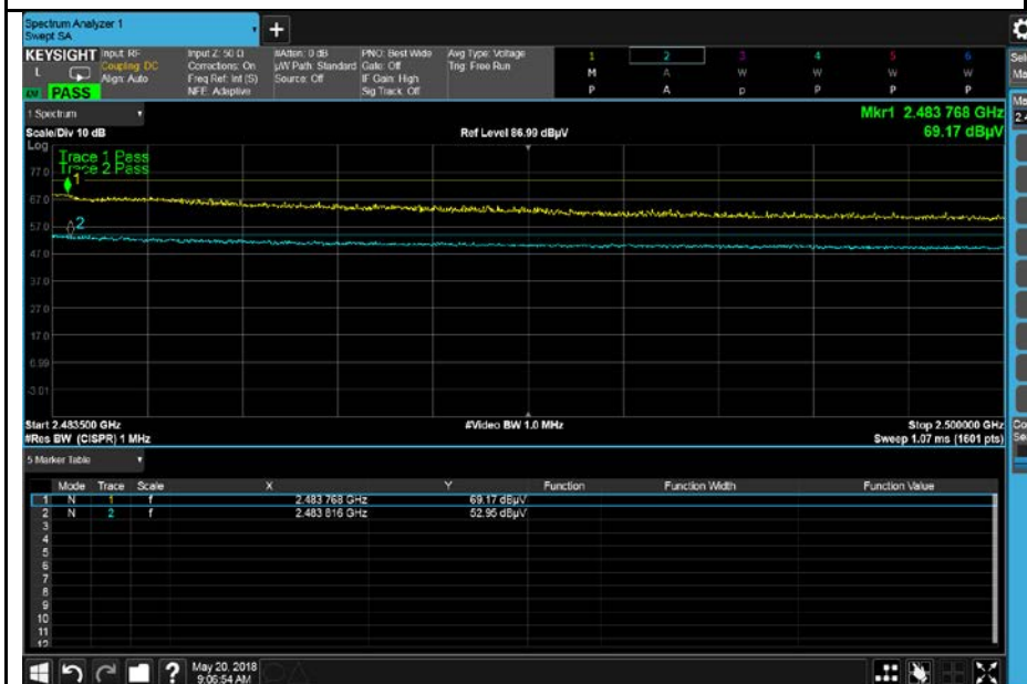
802.11n-HT20-2462MHz
