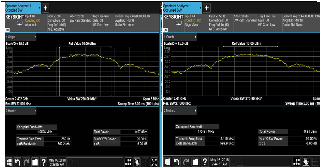
6dB BW –Bluetooth LE 2402MHz
