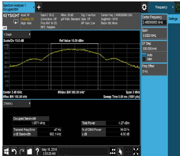
6dB BW –Bluetooth LE 2480MHz
