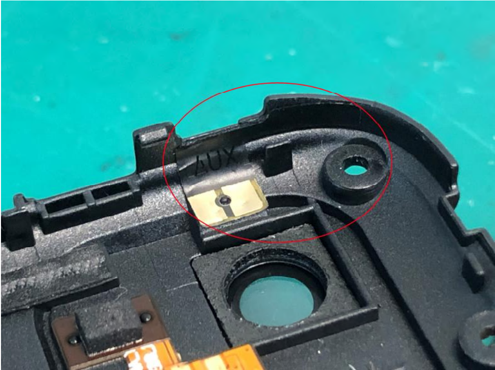
Antenna-AUX
