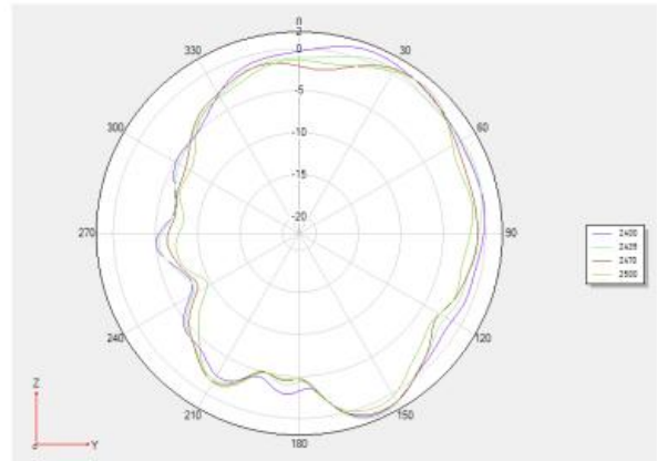
Phi 90 2D图
