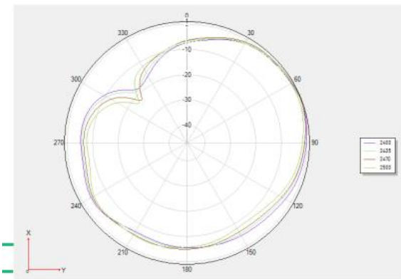
Theta 90 2D图
