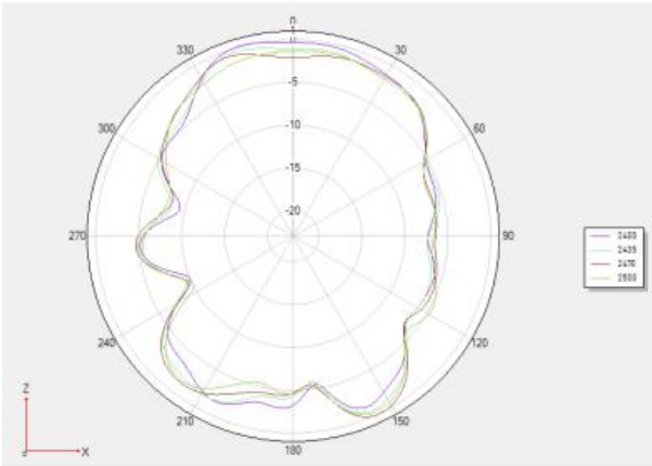
Phi 0 2D图
