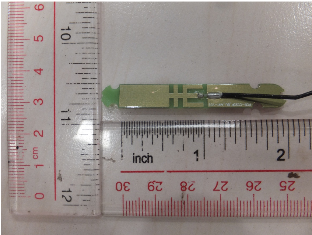
Fig. 6. Wi-Fi antenna
