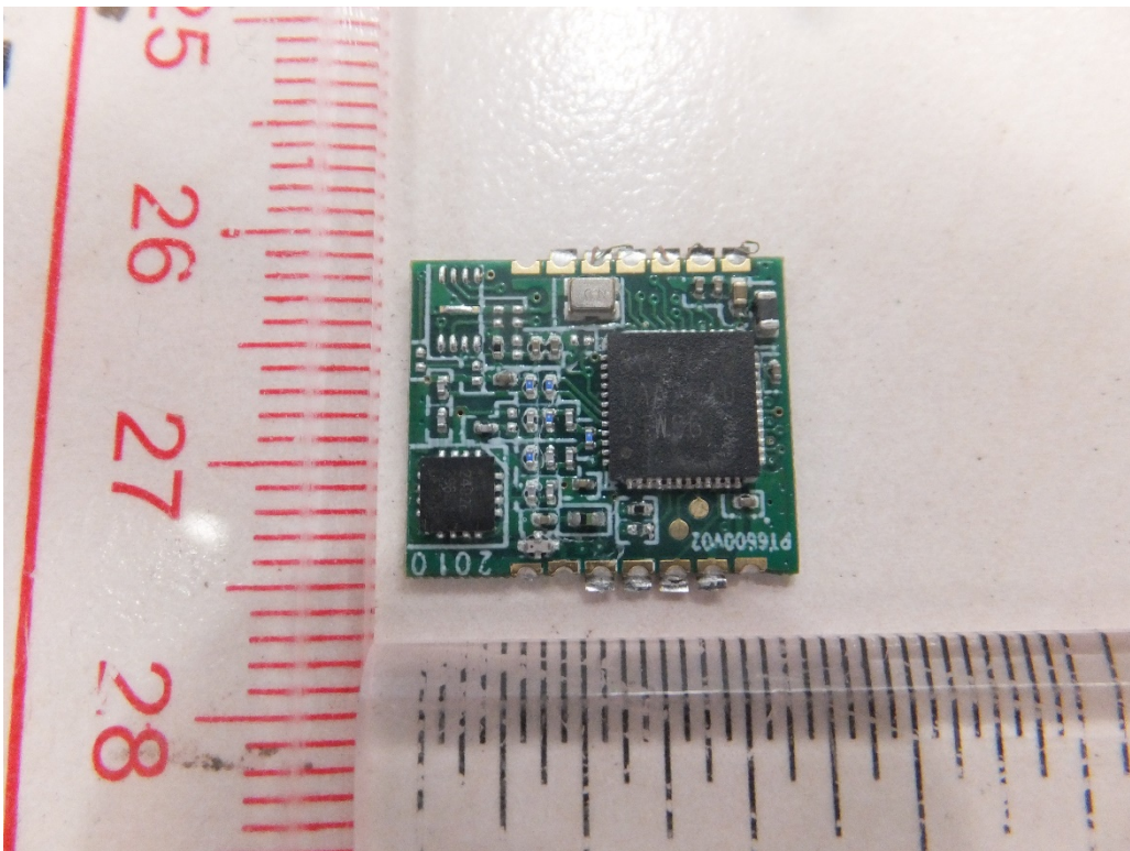
Fig. 8. Wi-Fi module
