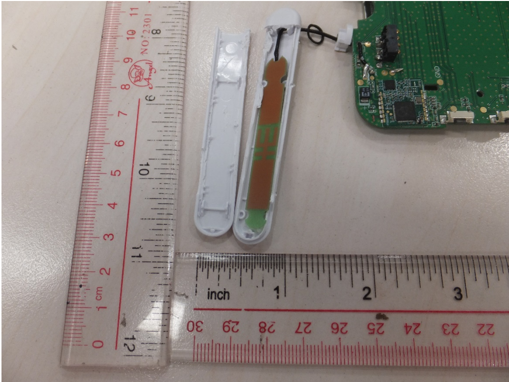
Fig. 5. Wi-Fi antenna
