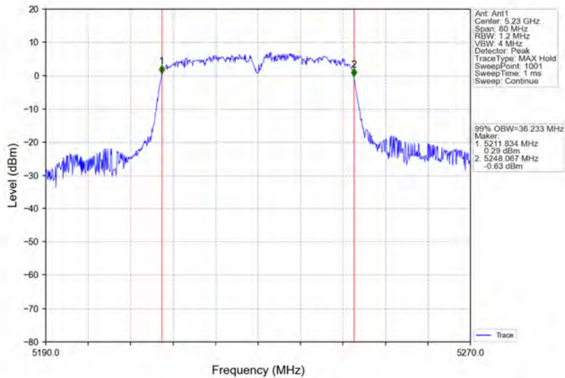
802.11n(HT40)_HCH_5230MHz_Ant1_NTNV
