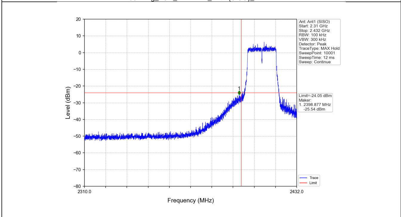
802.11g_LCH_2412MHz_Ant1 (SISO)_NTNV
