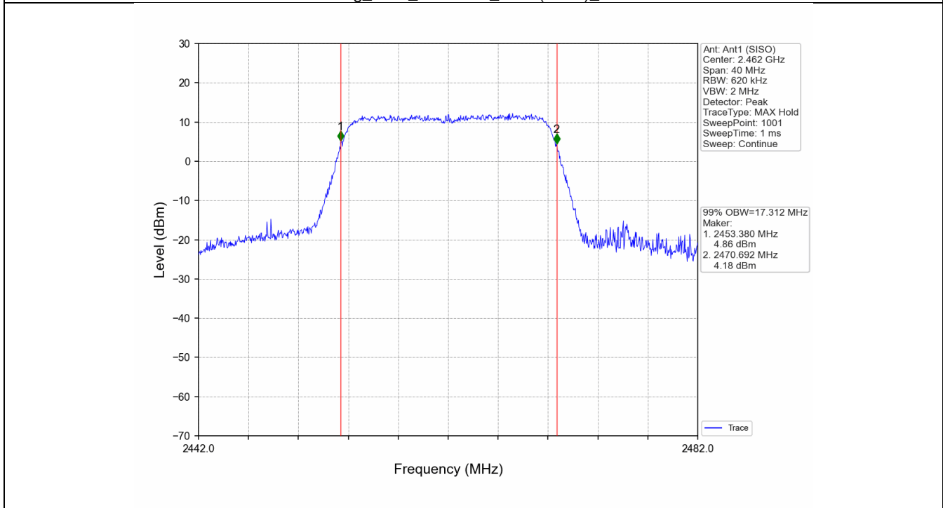
802.11g_HCH_2462MHz_Ant1 (SISO)_NTNV
