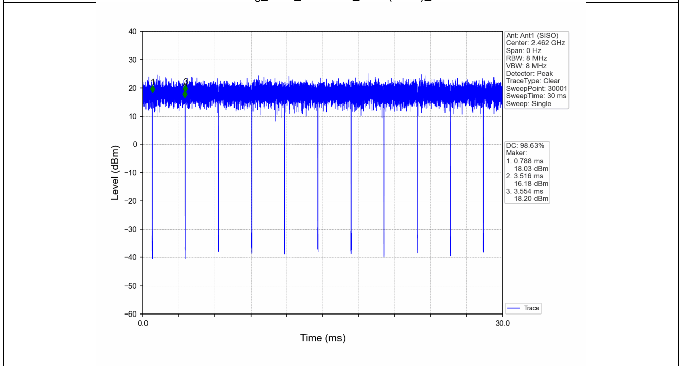
802.11g_HCH_2462MHz_Ant1 (SISO)_NTNV
