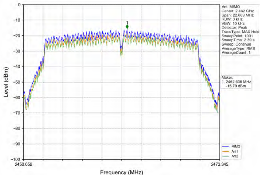
802.11n(HT20)_HCH_2462MHz_MIMO_NTNV
