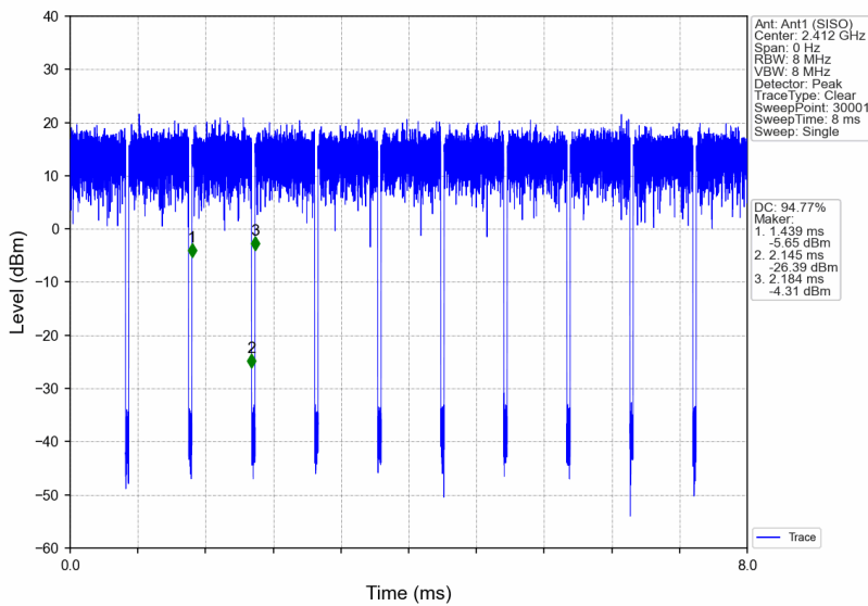
802.11g_LCH_2412MHz_Ant1 (SISO)_NTNV
