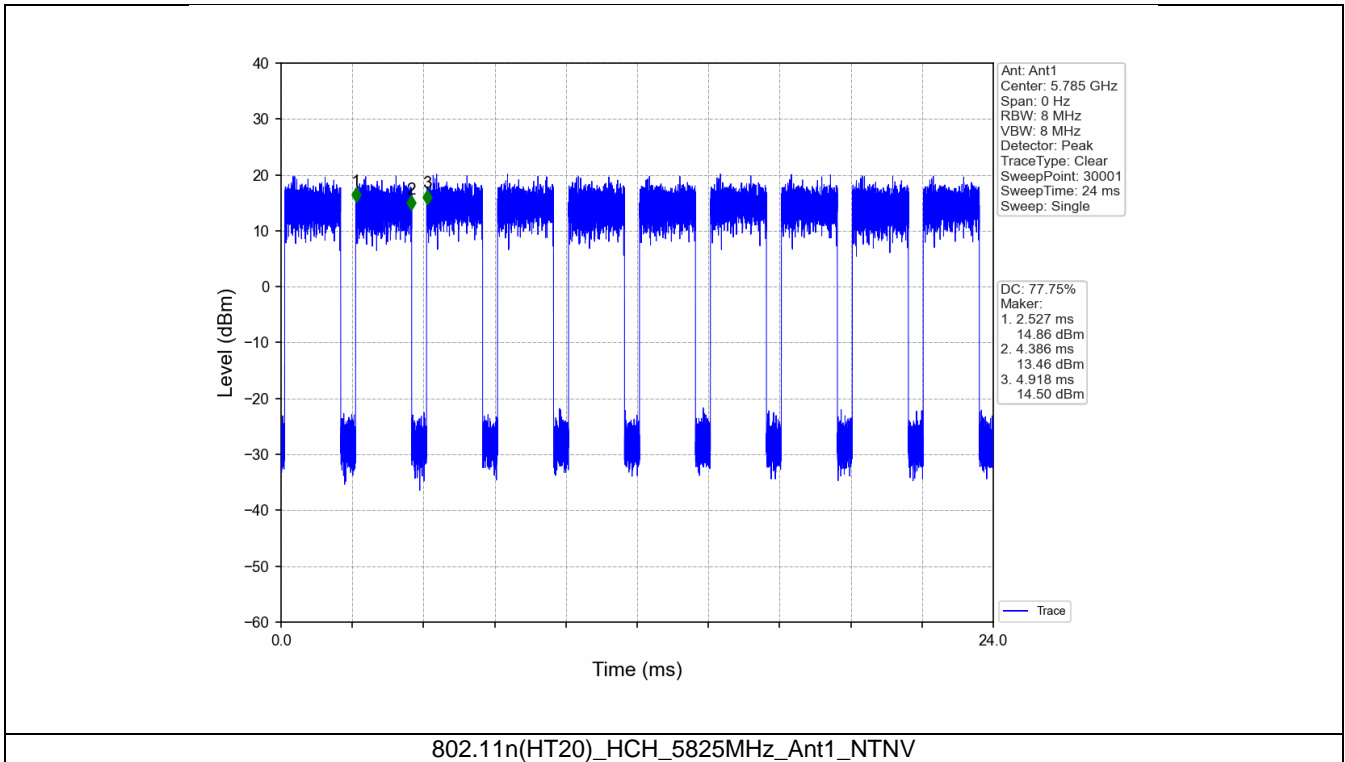
802.11n(HT20)_HCH_5825MHz_Ant1_NTNV
