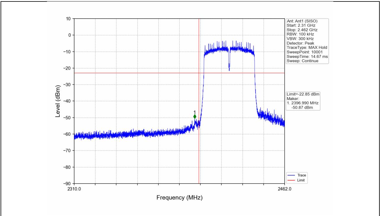
802.11n(HT40)_LCH_2422MHz_Ant1 (SISO)_NTNV
