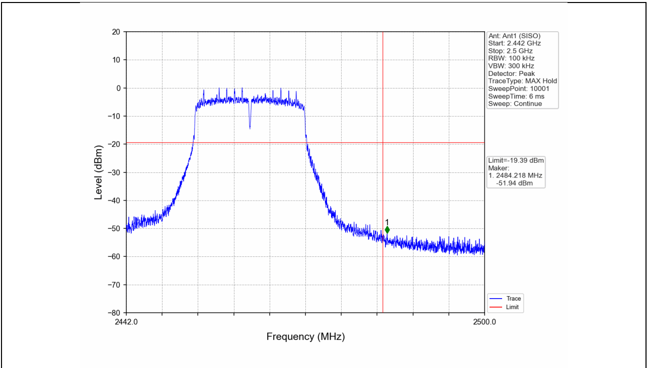
802.11n(HT20)_HCH_2462MHz_Ant1 (SISO)_NTNV
