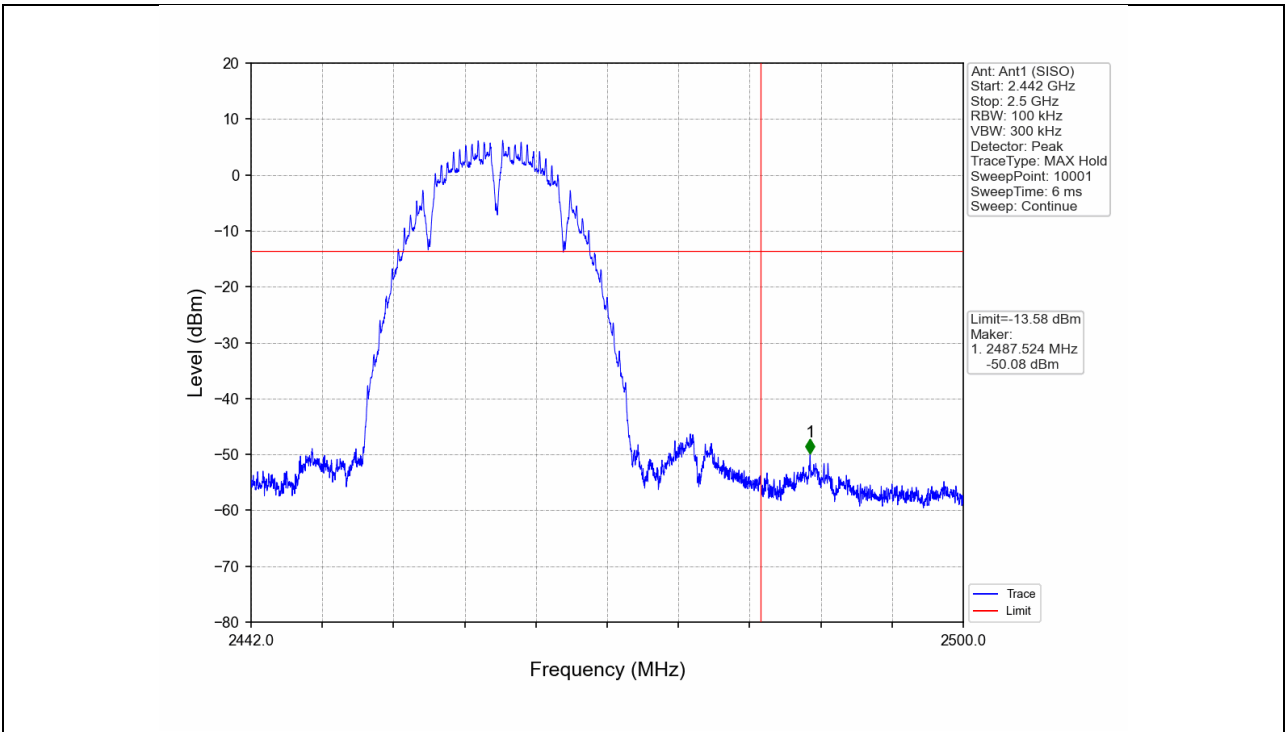
802.11b_HCH_2462MHz_Ant1 (SISO)_NTNV
