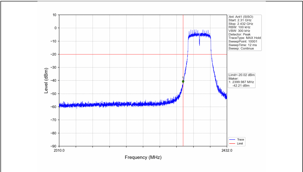
802.11g_LCH_2412MHz_Ant1 (SISO)_NTNV
