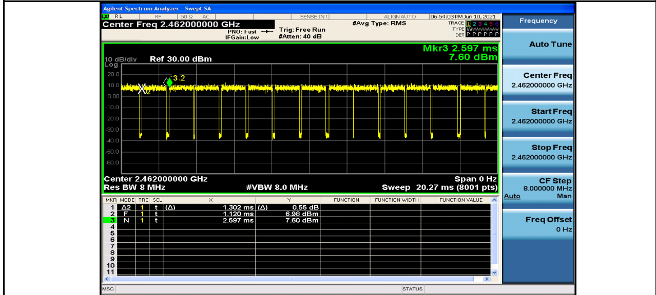
Duty Cycle_11N20MIMO_2462_Ant2
