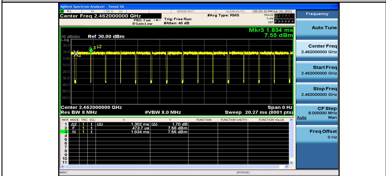
Duty Cycle_11N20MIMO_2462_Ant2
