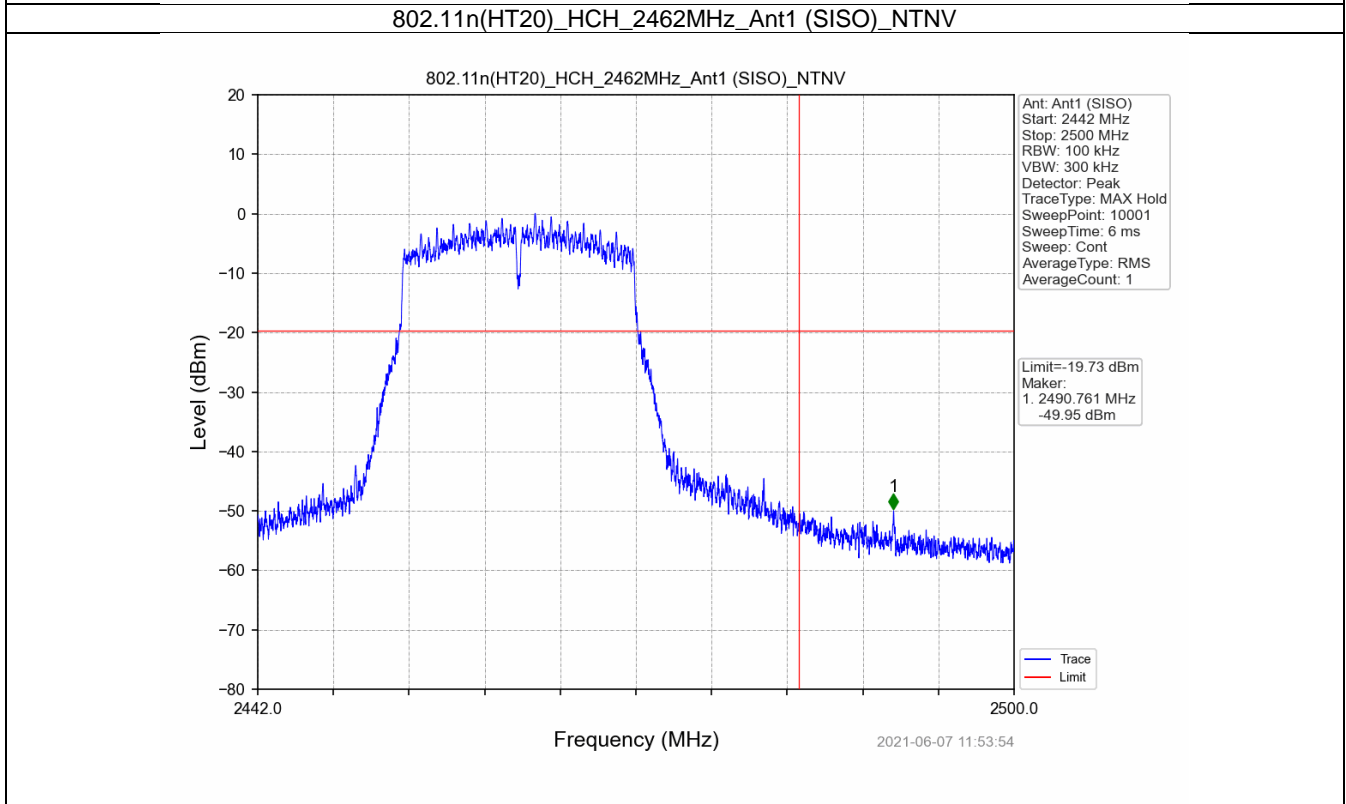
802.11n(HT20)_HCH_2462MHz_Ant1 (SISO)_NTNV
