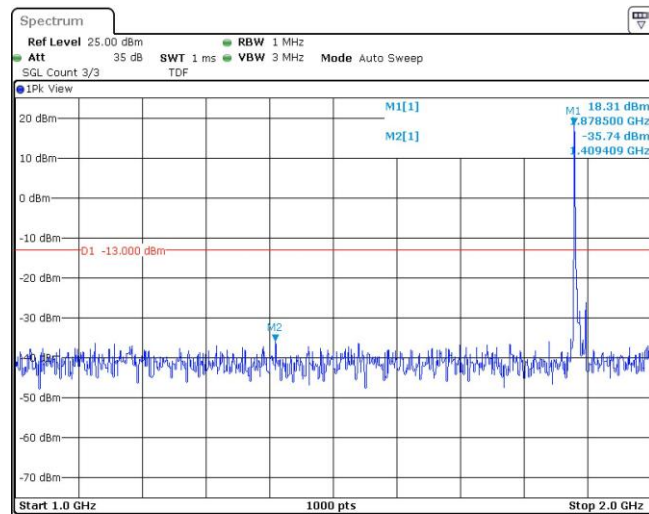
Band25-10MHz-QPSK-26365-1RB#0-Range3:2000~20000MHz
