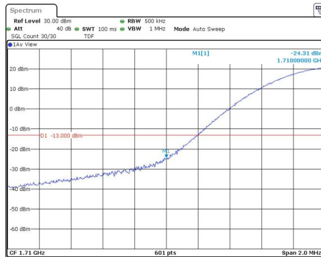
Band66-20MHz-QPSK-132072-1RB#99
