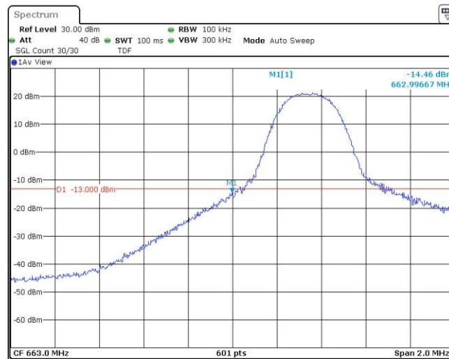
Band71-5MHz-QPSK-133147-1RB#24
