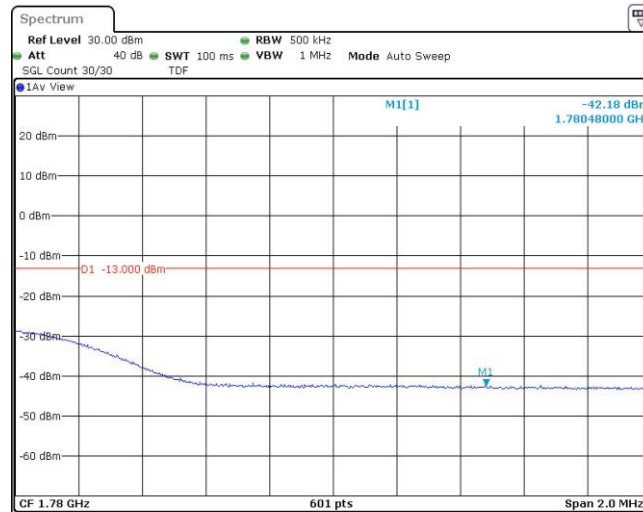
Band66-20MHz-QPSK-132572-1RB#99
