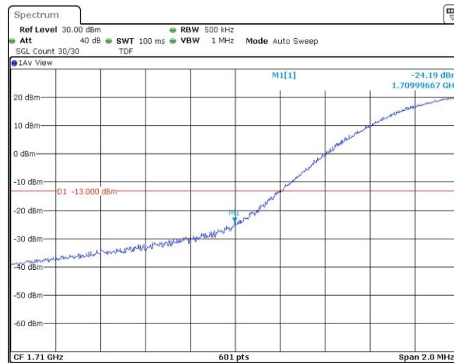
Band66-20MHz-16QAM-132072-1RB#99
