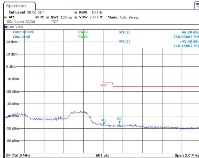
Band12-3MHz-QPSK-23165-1RB#14
