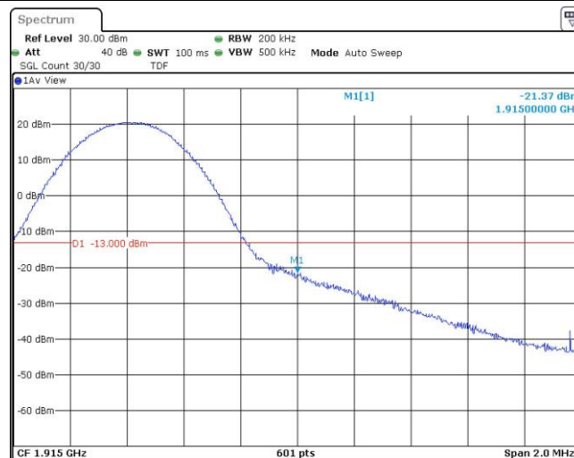
Band25-10MHz-QPSK-26640-50RB#0
