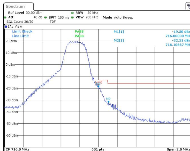
Band12-3MHz-QPSK-23165-15RB#0
