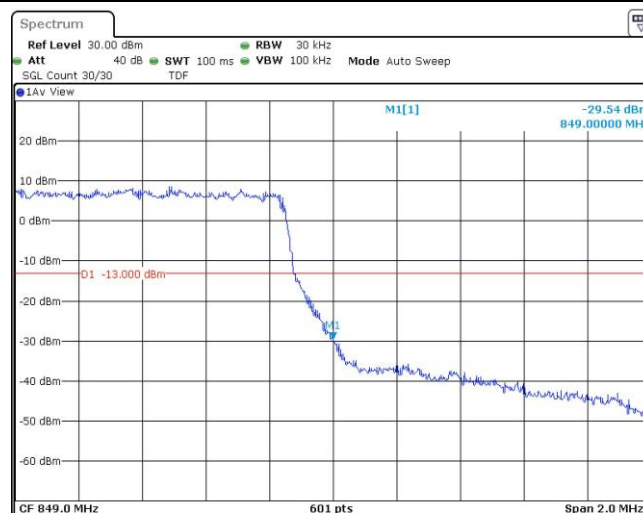
Band5-3MHz-QPSK-20415-1RB#0
