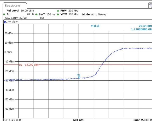
Band4-10MHz-QPSK-20350-1RB#0
