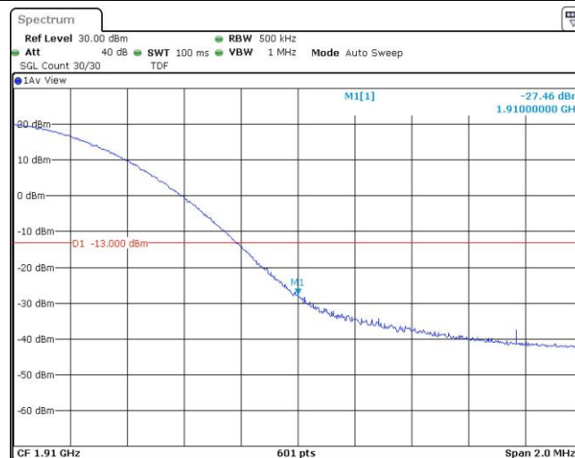
Band2-20MHz-16QAM-19100-100RB#0
