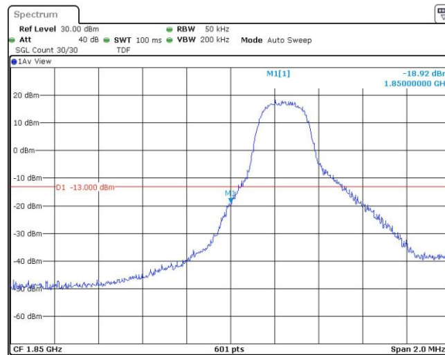
Band2-3MHz-QPSK-18615-1RB#14
