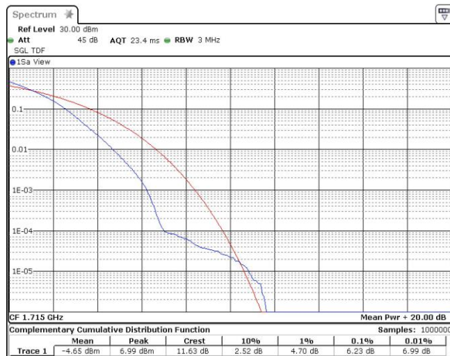
Band66-10MHz-QPSK-132022-50RB#0
