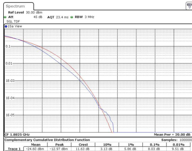
Band25-20MHz-QPSK-26365-100RB#0
