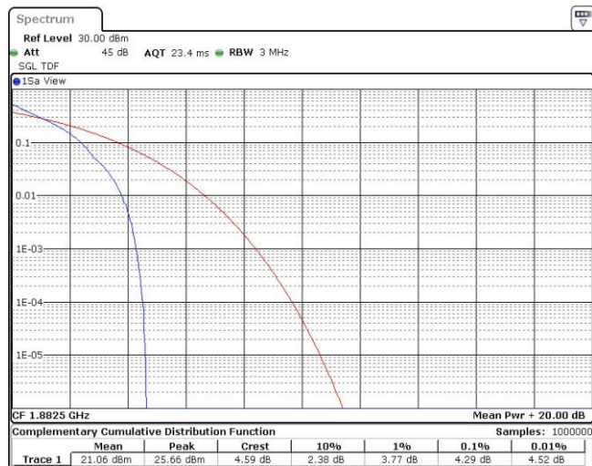
Band25-1.4MHz-QPSK-26365-6RB#0
