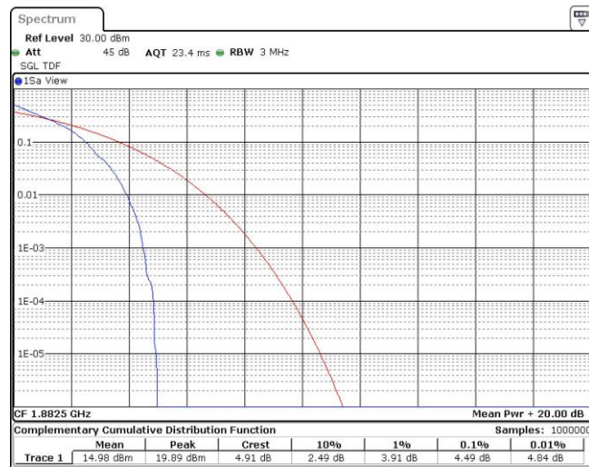
Band25-5MHz-QPSK-26365-25RB#0
