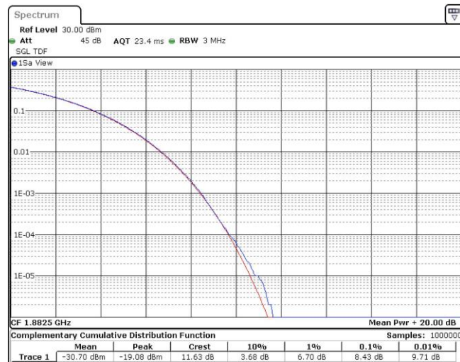
Band25-10MHz-QPSK-26365-50RB#0
