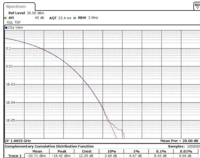
Band25-10MHz-16QAM-26365-50RB#0
