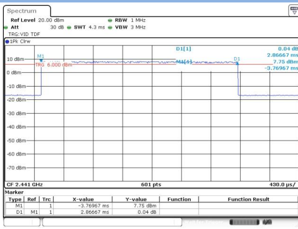
GFSK DH5
