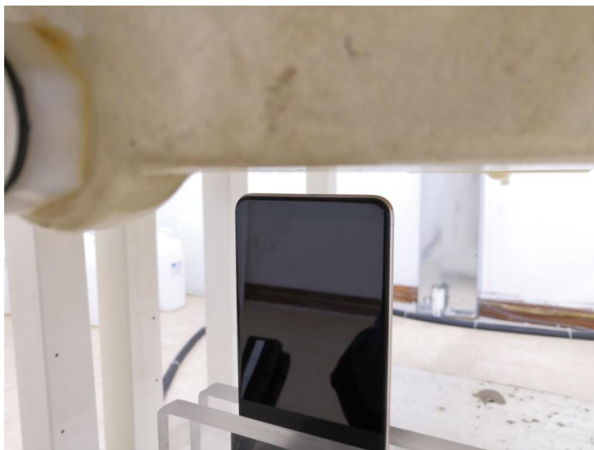
Top Side_10mm
