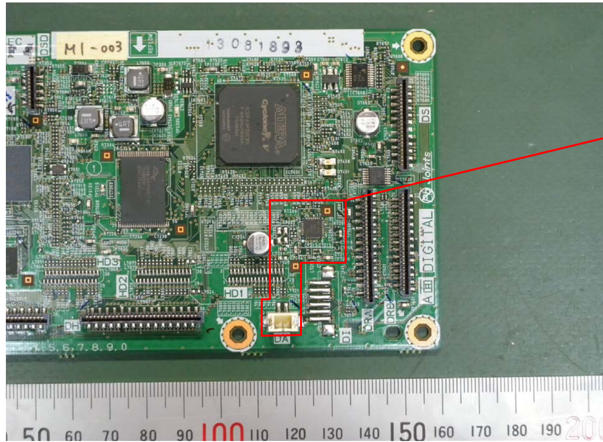
RFID Module
