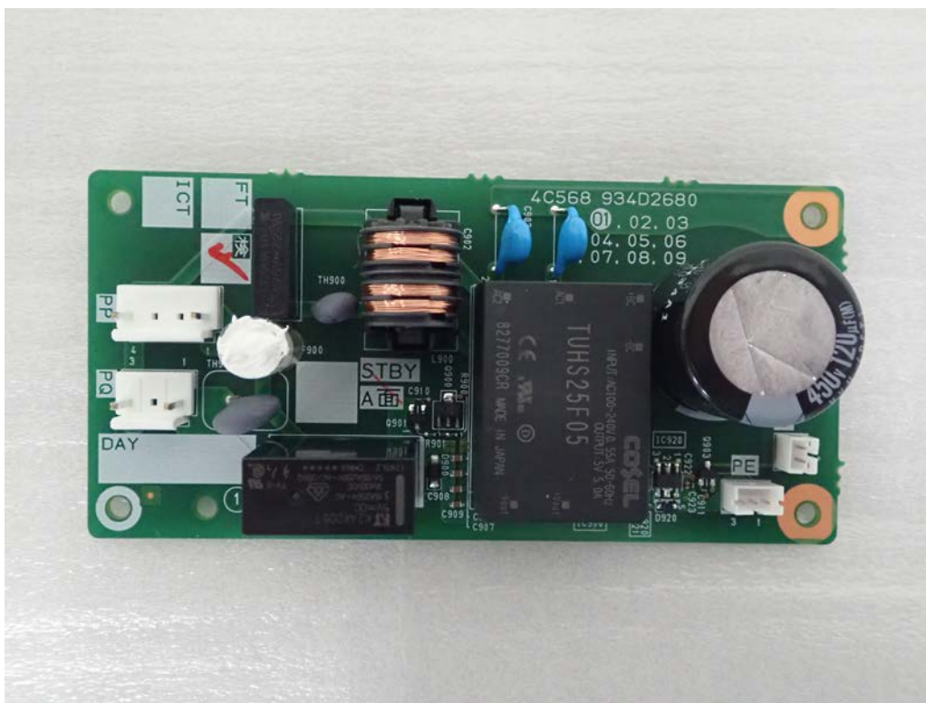
STBY-A
