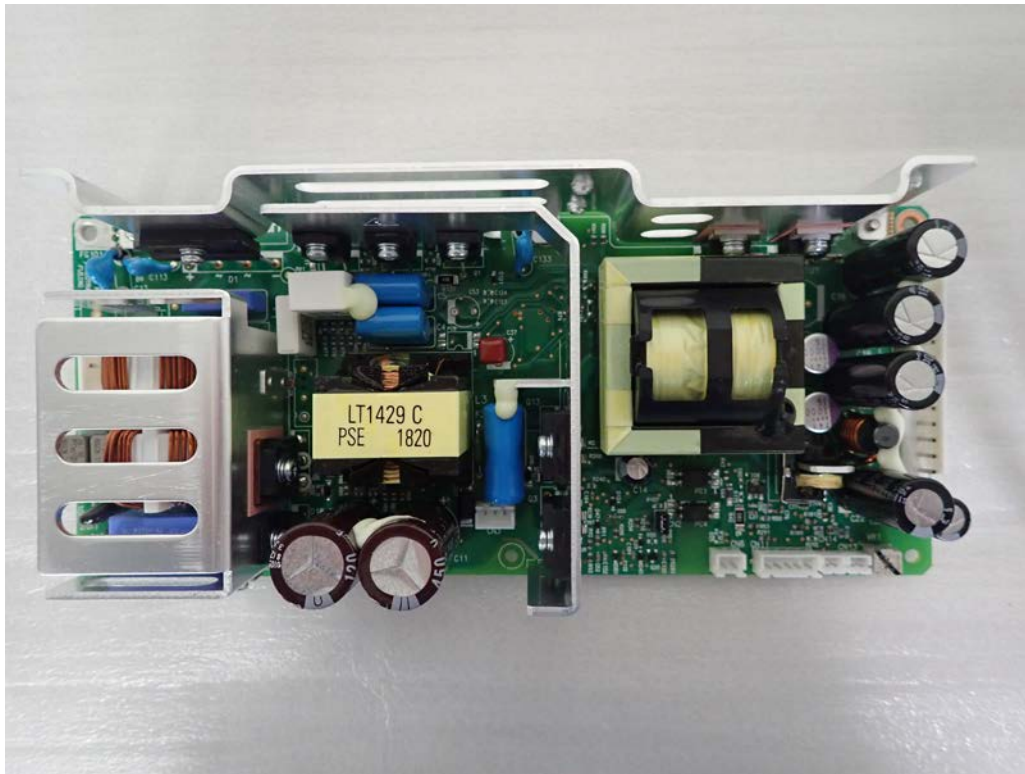
PSU-A
