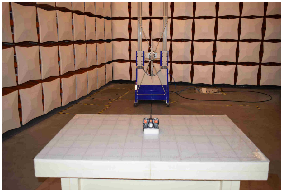
TX 30MHz ~1GHz
