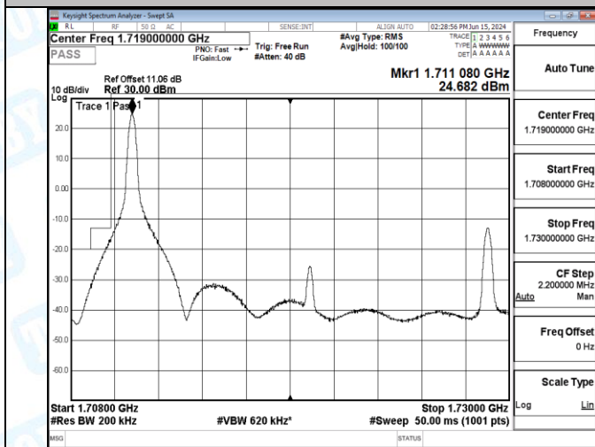
Band66_20MHz_QPSK_132072_100RB#0
