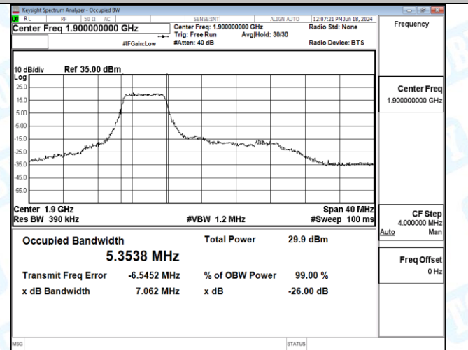
Band2-20MHz-16QAM-19100-27RB#0-PASS
