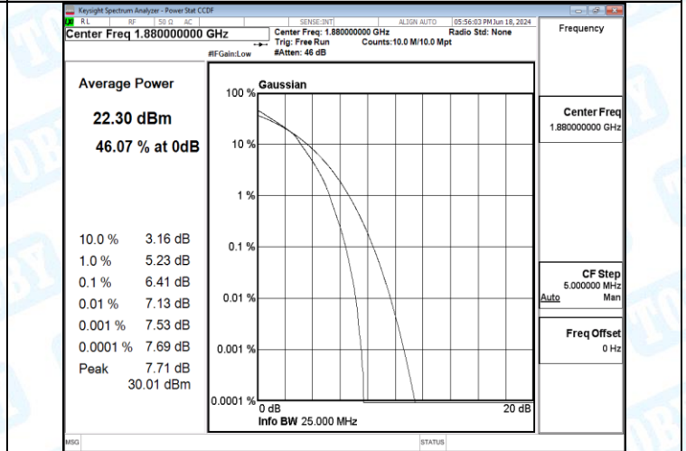
Band2-20MHz-16QAM-19100-27RB#0-PASS
