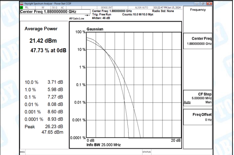
Band2-20MHz-QPSK-19100-100RB#0-PASS
