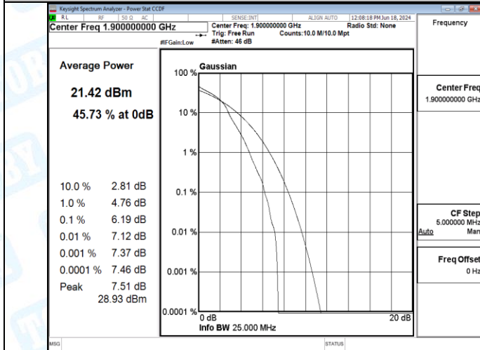
Band2-20MHz-16QAM-19100-1RB#0-PASS
