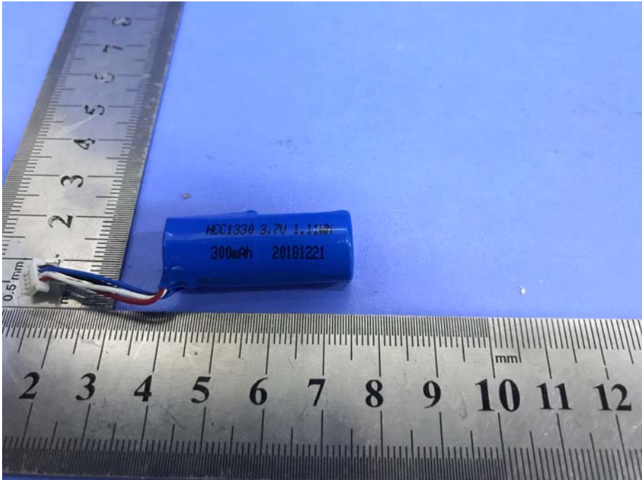
Photo 12 Battery parameter
