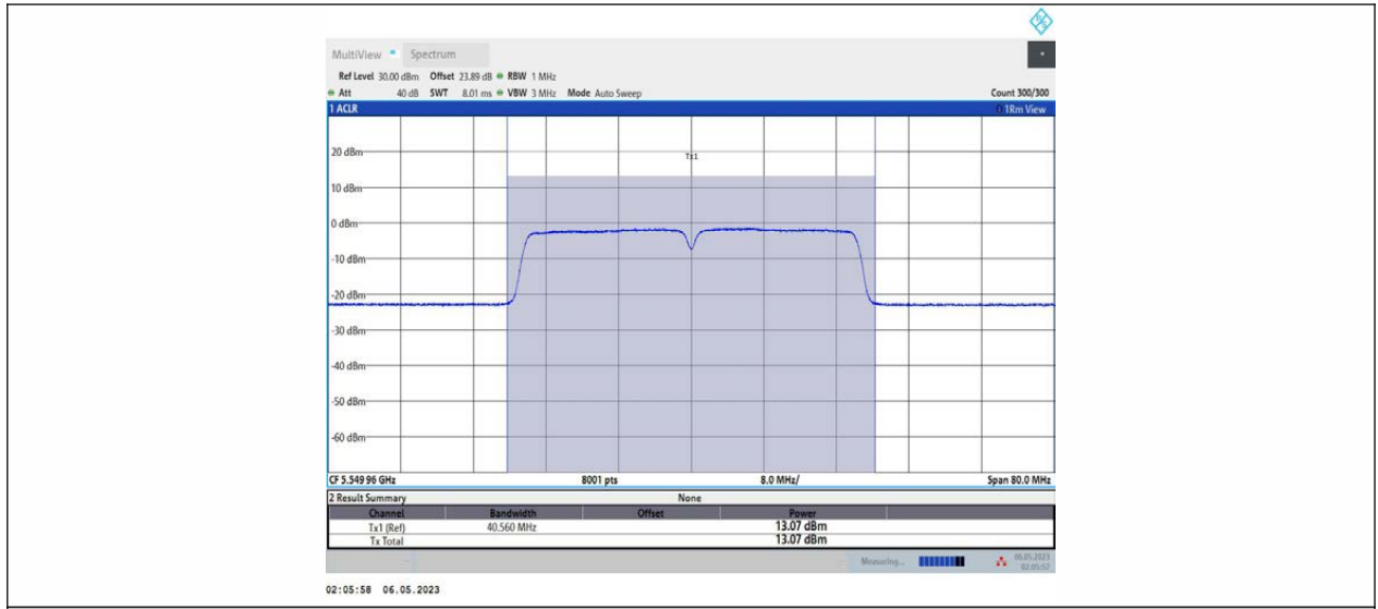
11AC40MIMO_Ant2_5550
