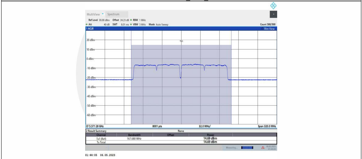
11AC160MIMO_Ant2_5570
