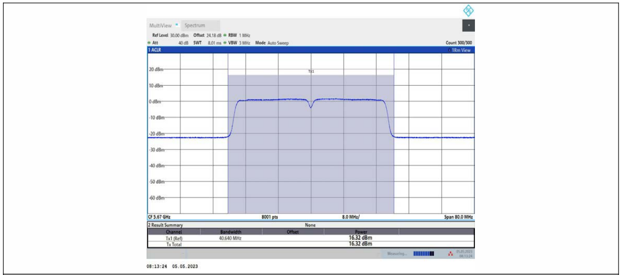
11AC40MIMO_Ant1_5670
