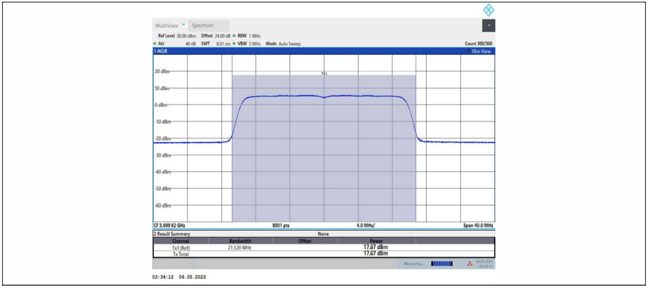
11AX20MIMO_Ant2_5700
