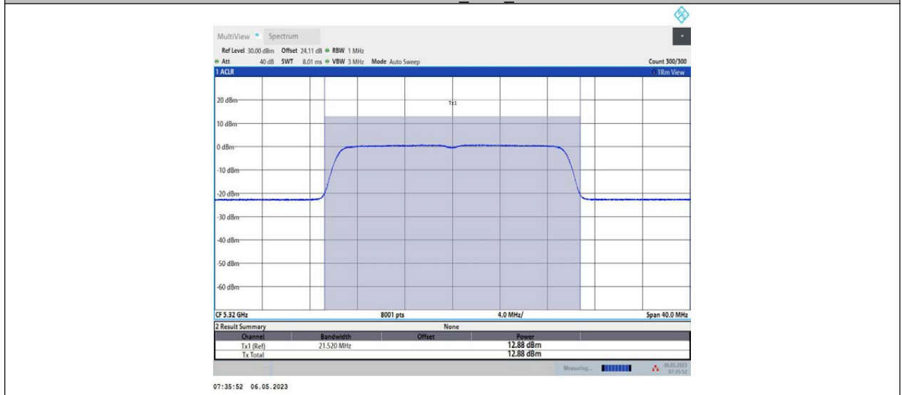
11AX20MIMO_Ant1_5320
