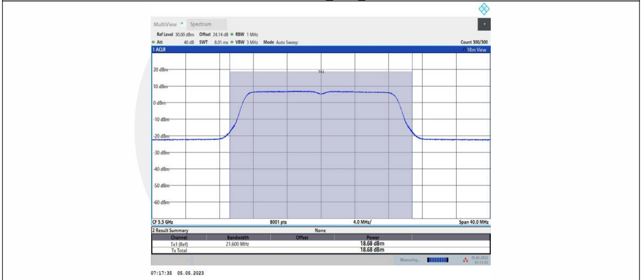
11AC20MIMO_Ant1_5500
