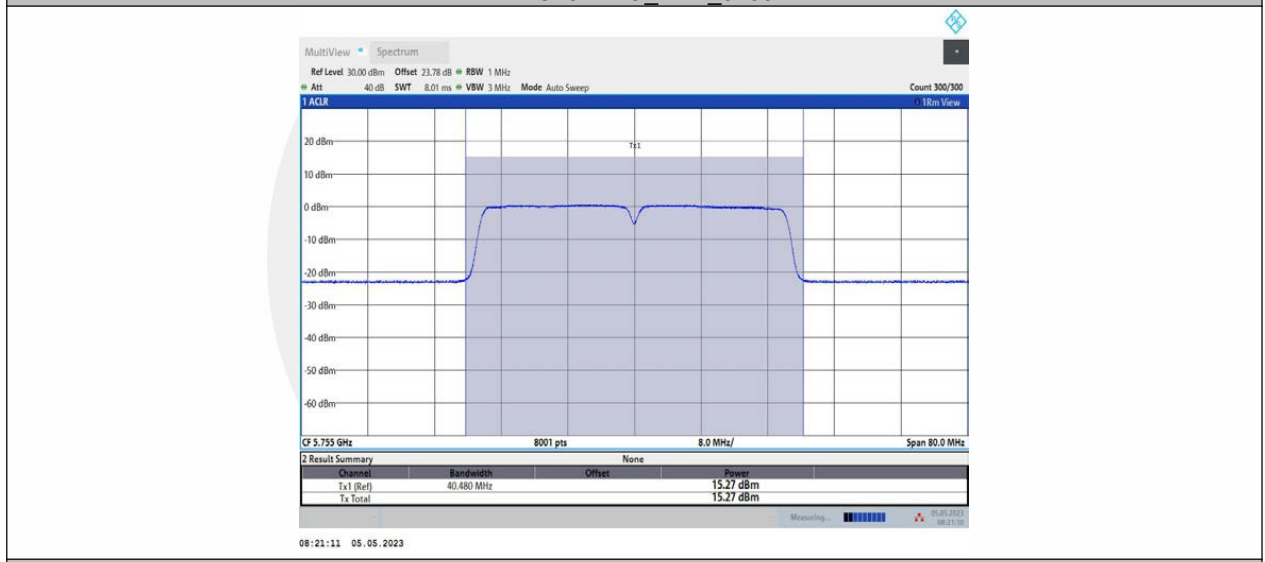
11AC40MIMO_Ant2_5755
