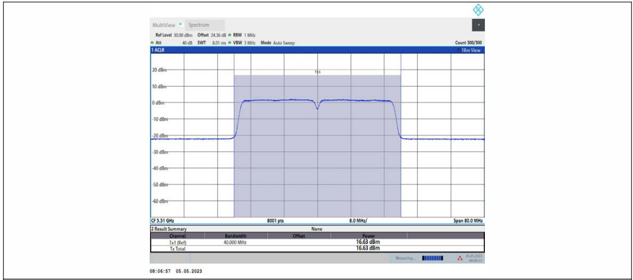
11AC40MIMO_Ant2_5510
