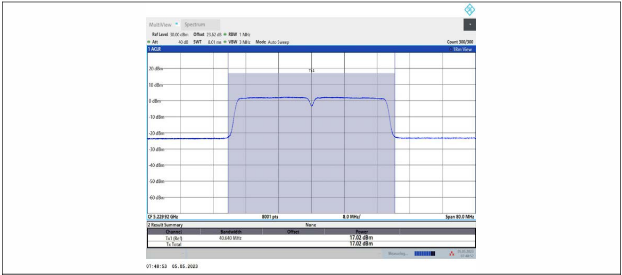
11AC40MIMO_Ant2_5230
