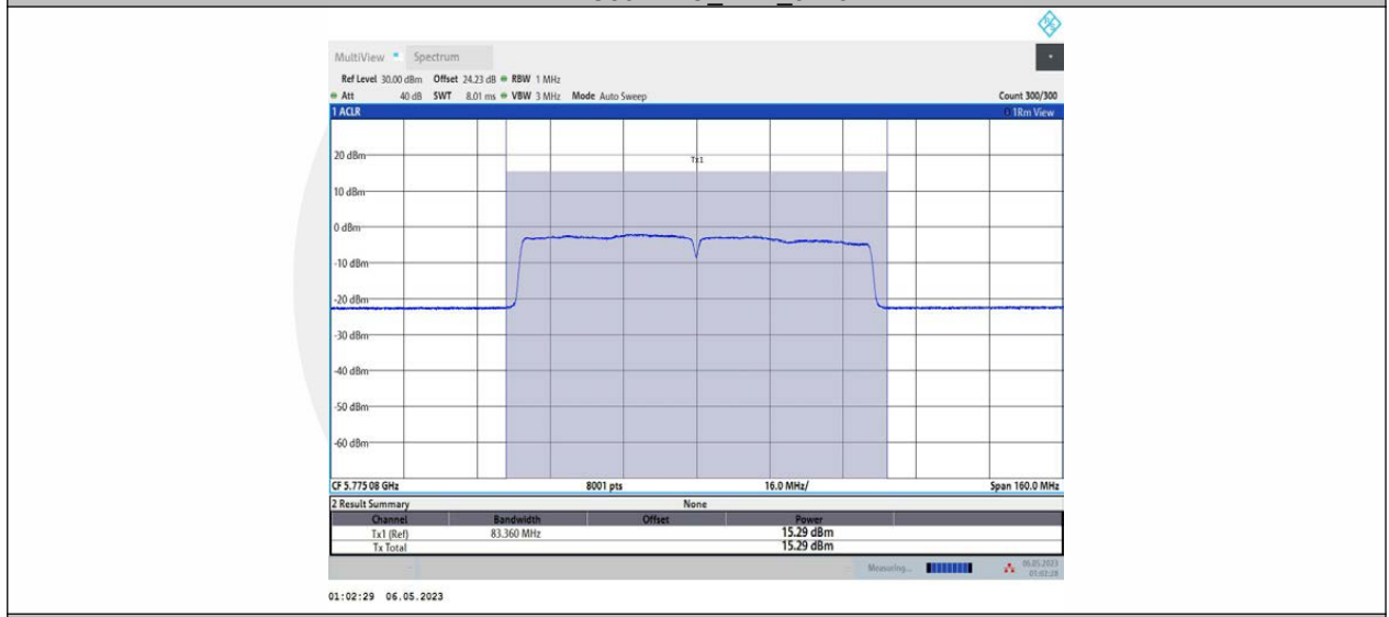
11AC80MIMO_Ant2_5775
