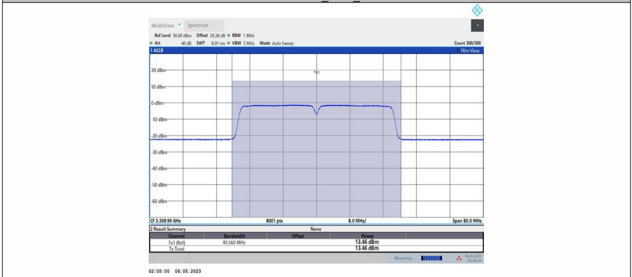
11AC40MIMO_Ant2_5510
