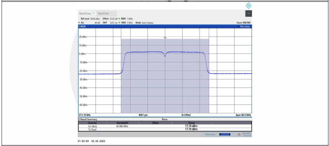
11AC40MIMO_Ant2_5190
