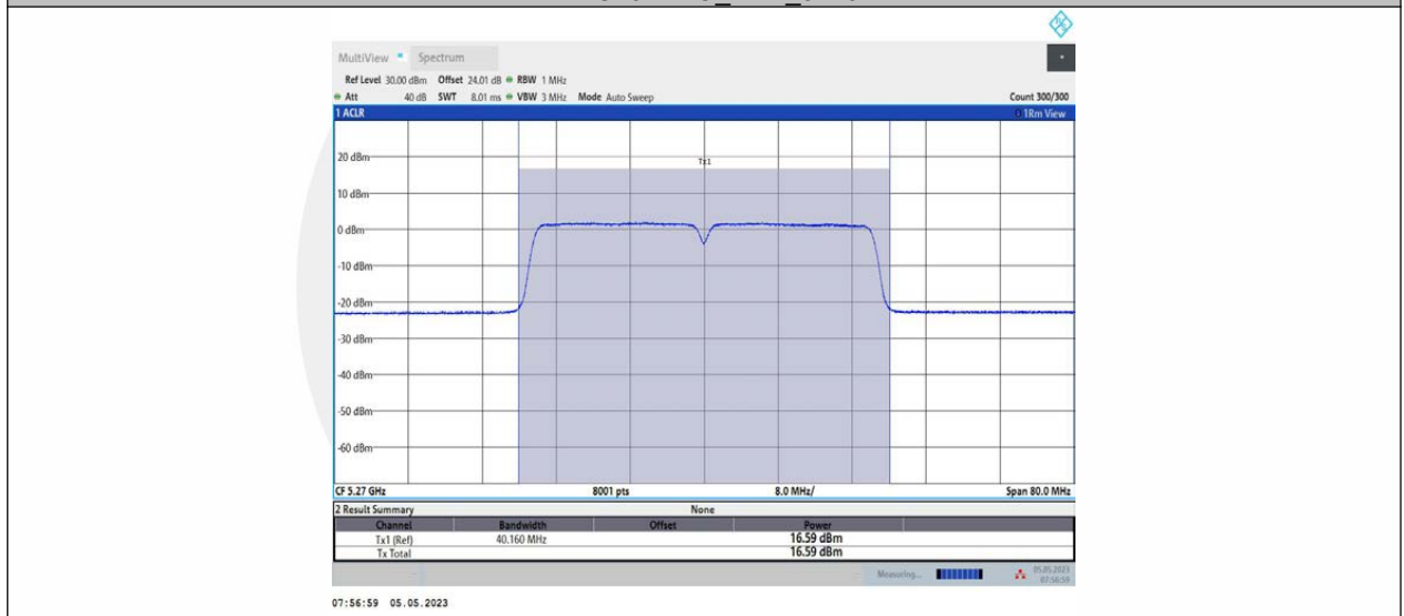
11AC40MIMO_Ant2_5270
