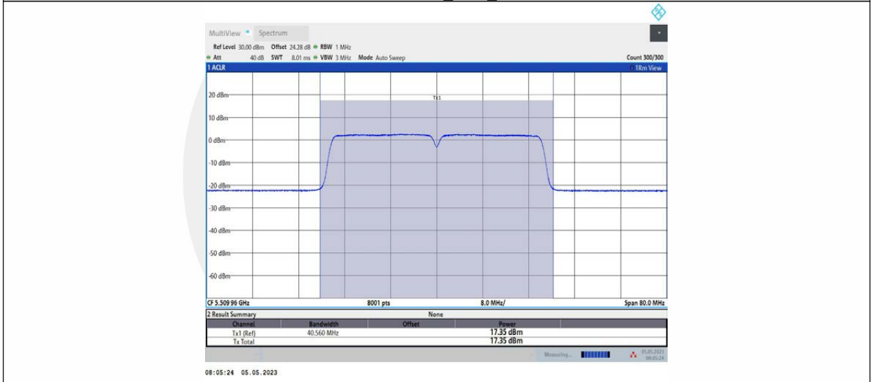
11AC40MIMO_Ant1_5510
