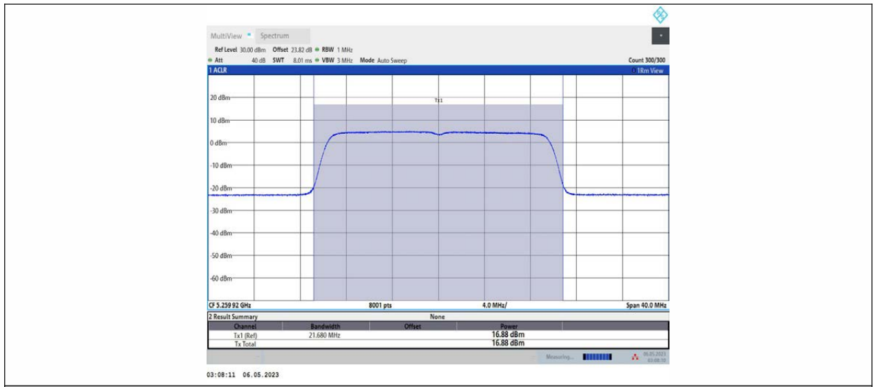
11AX20MIMO_Ant1_5260
