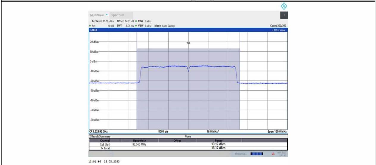
11AC80MIMO_Ant1_5530
