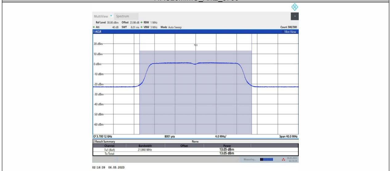
11AC20MIMO_Ant2_5700
