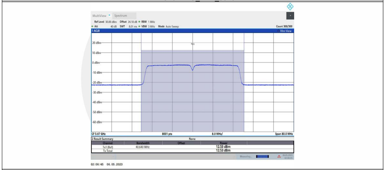
11AC40MIMO_Ant2_5670
