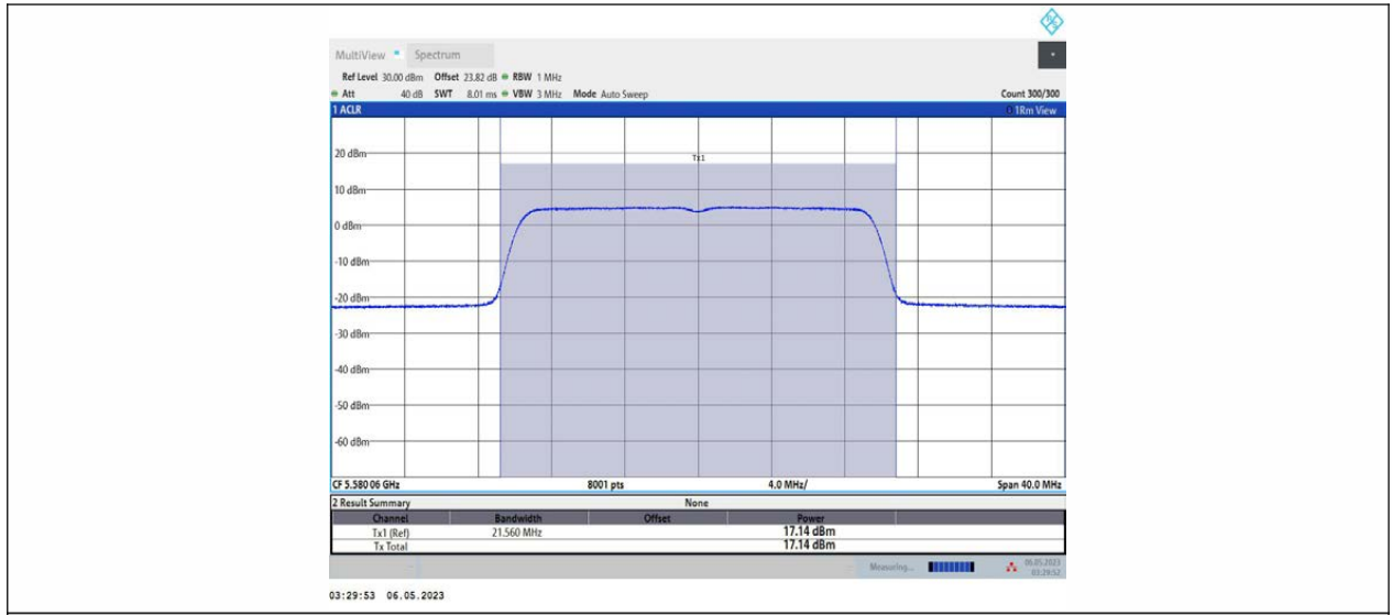
11AX20MIMO_Ant2_5580
