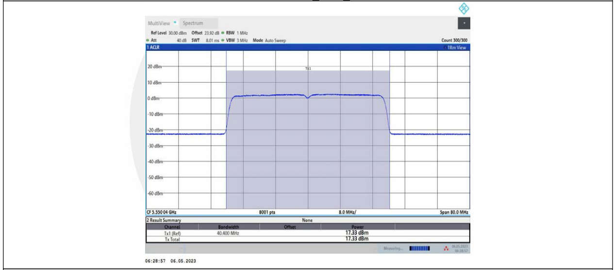
11AX40MIMO_Ant1_5550
