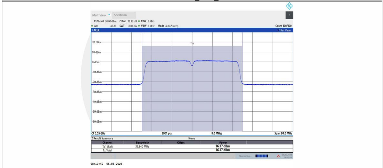
11AC40MIMO_Ant2_5550
