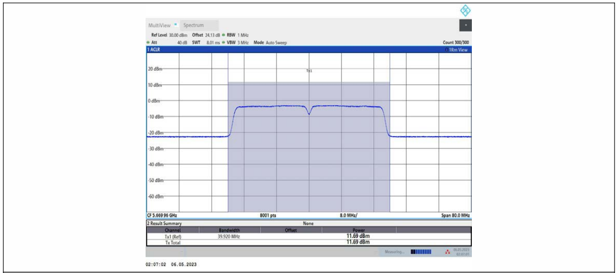
11AC40MIMO_Ant1_5755
