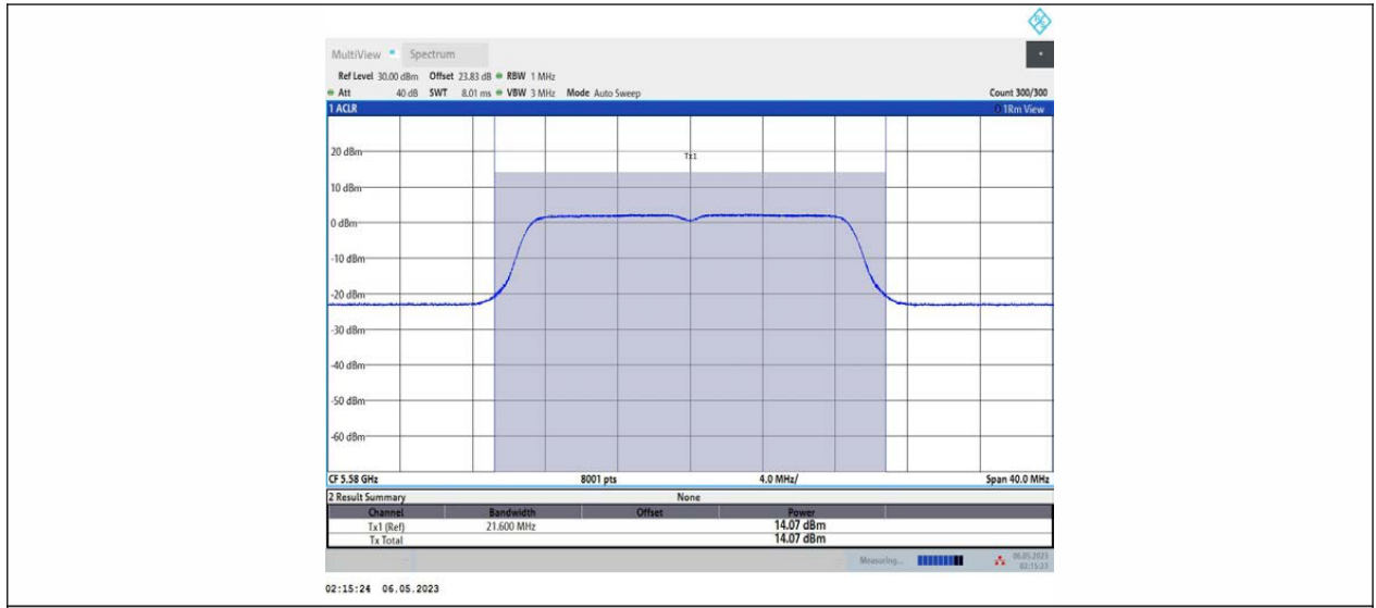
11AC20MIMO_Ant2_5580
