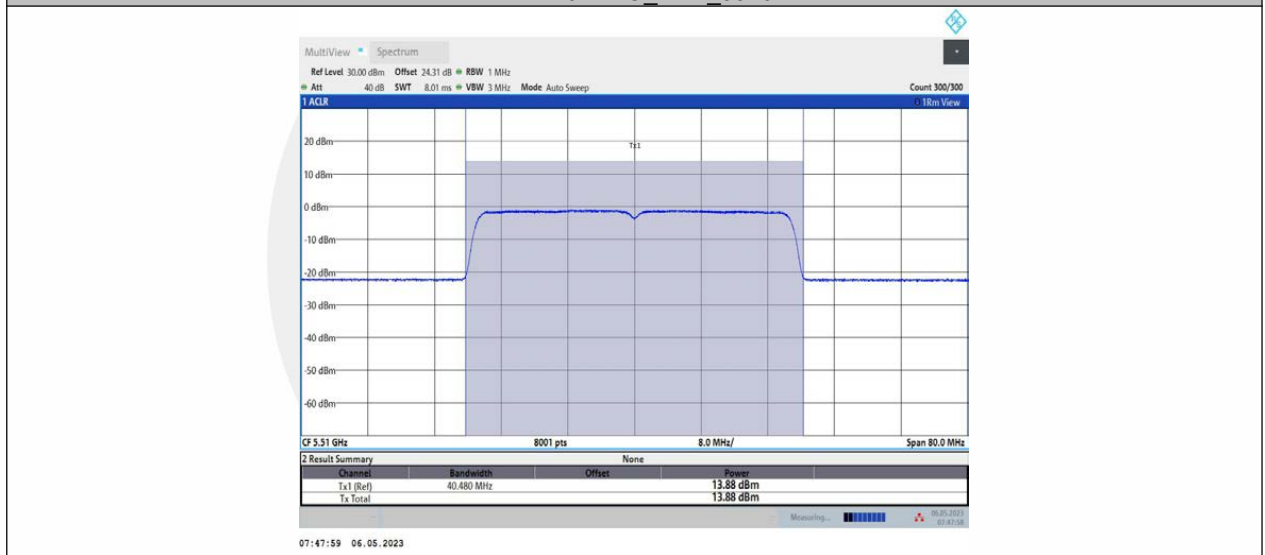
11AX40MIMO_Ant2_5510
