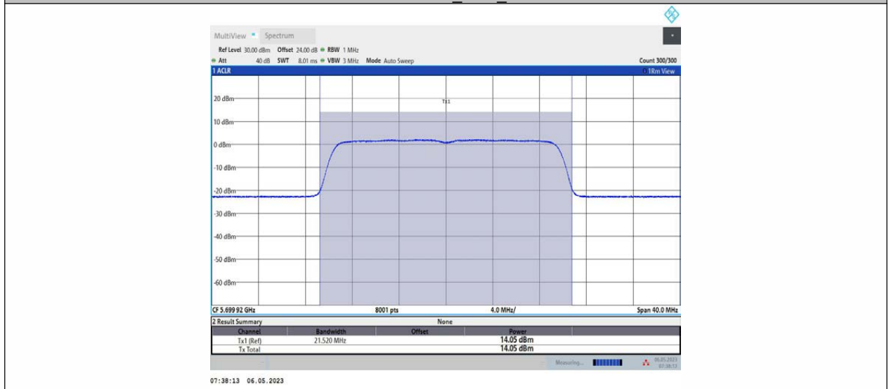
11AX20MIMO_Ant1_5700
