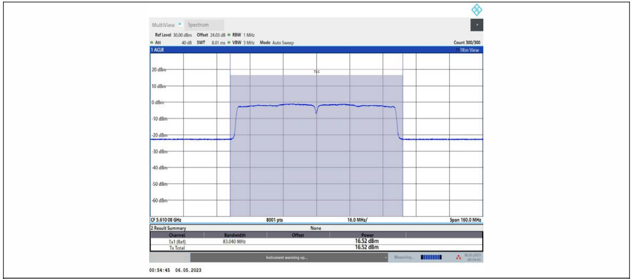
11AC80MIMO_Ant1_5610
