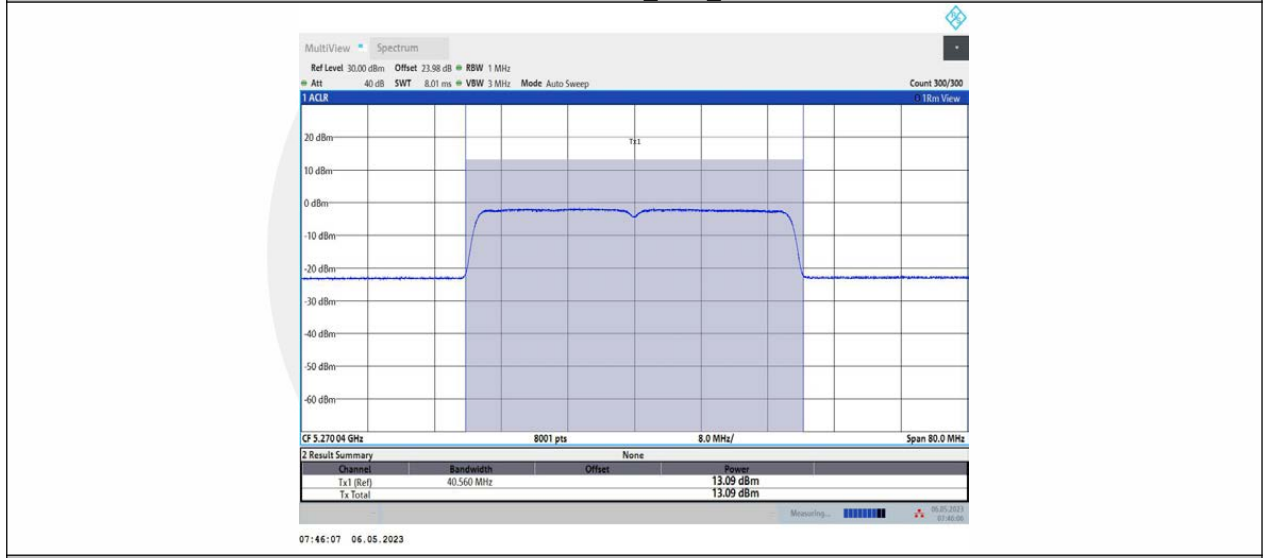
11AX40MIMO_Ant1_5270
