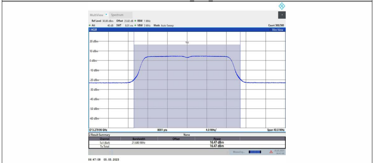
11AC20MIMO_Ant1_5280
