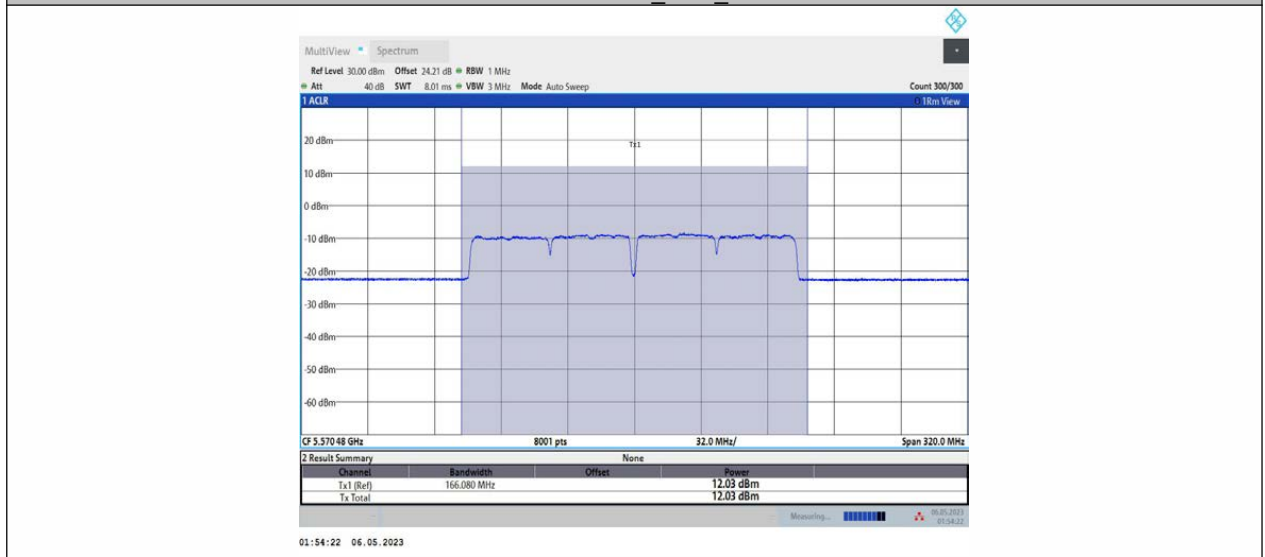
11AC160MIMO_Ant1_5570
