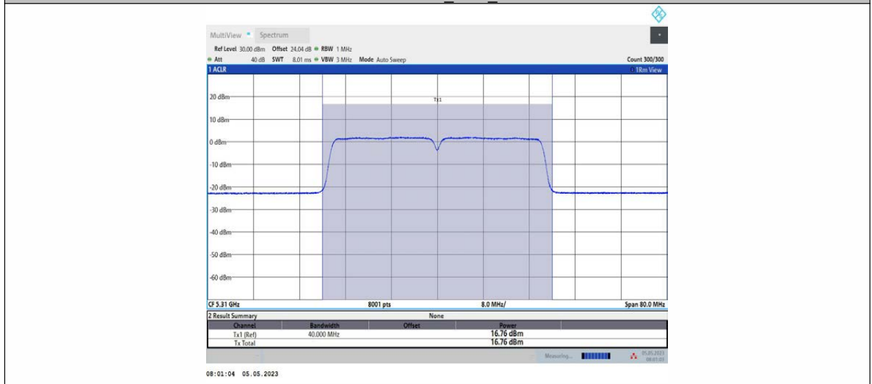
11AC40MIMO_Ant2_5310
