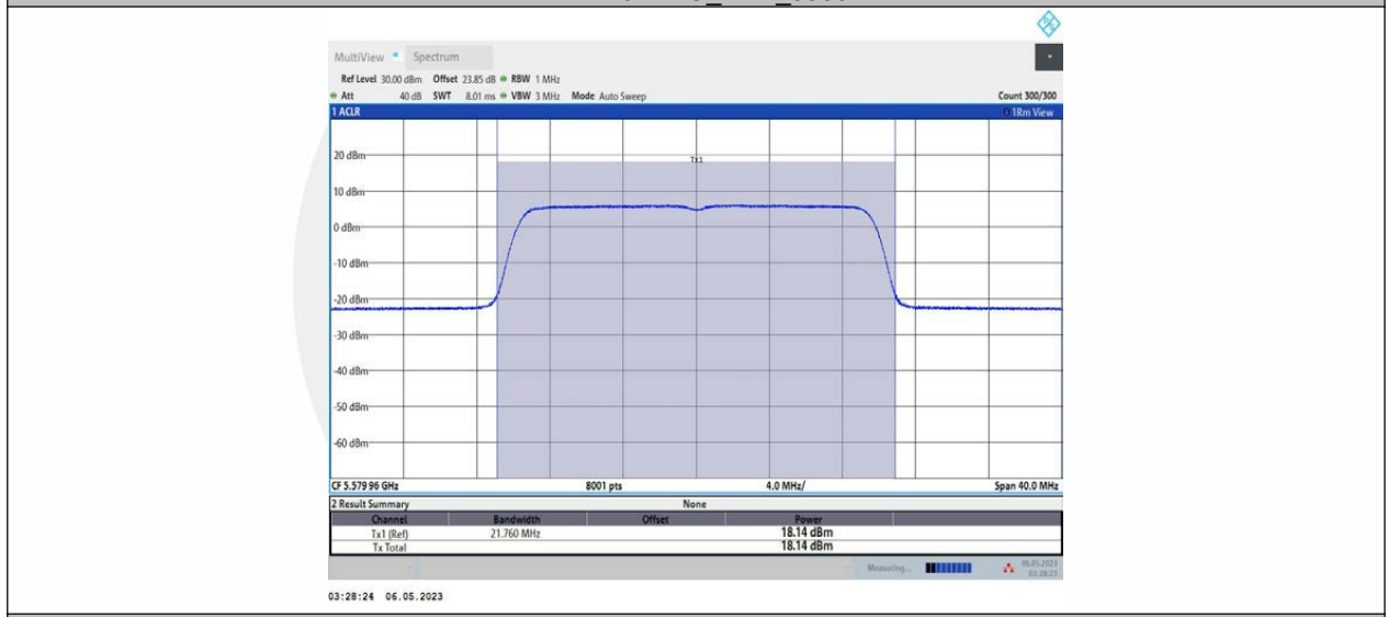
11AX20MIMO_Ant1_5580
