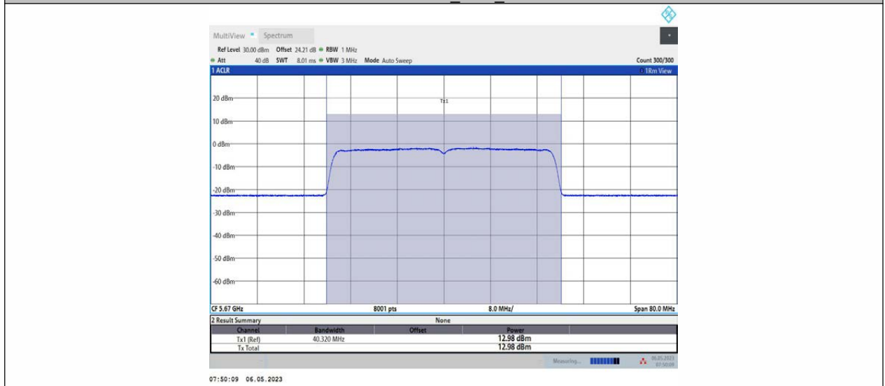
11AX40MIMO_Ant1_5670
