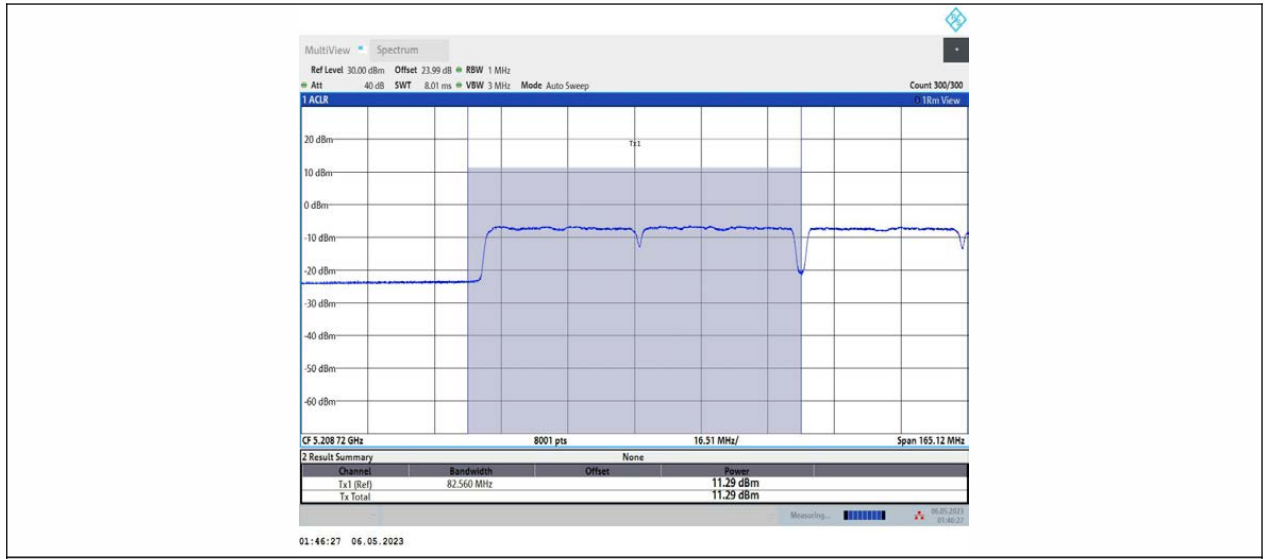
11AC160MIMO_Ant1_5250_UNII-1
