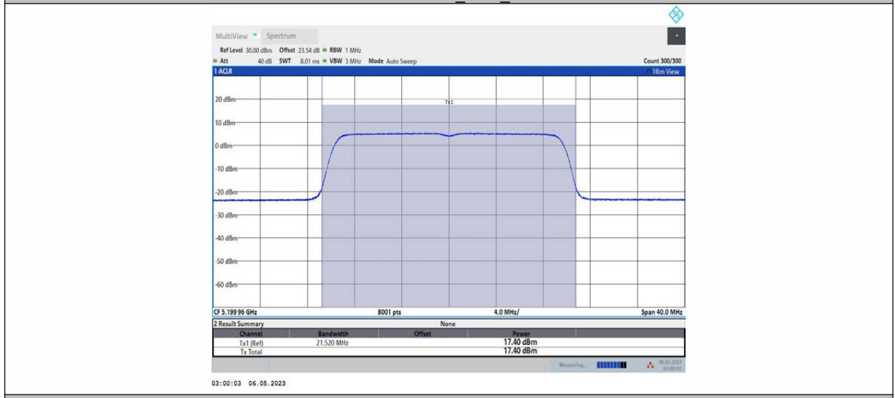
11AX20MIMO_Ant2_5200
