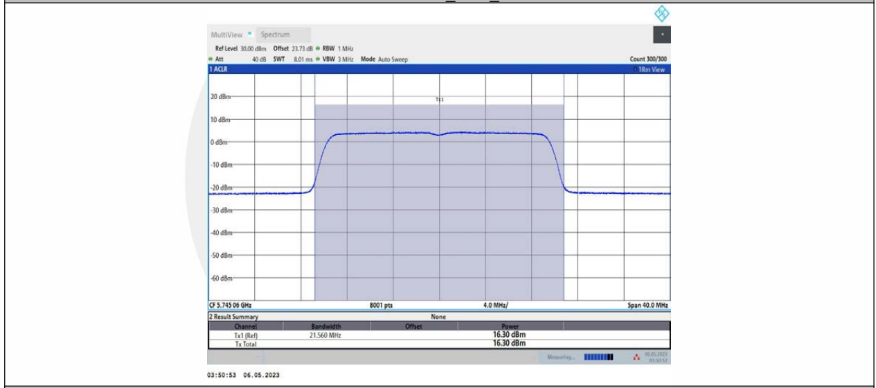
11AX20MIMO_Ant1_5785
