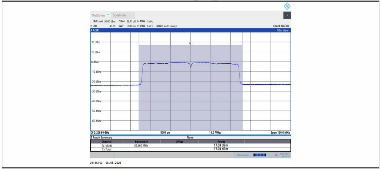
11AC80MIMO_Ant2_5210
