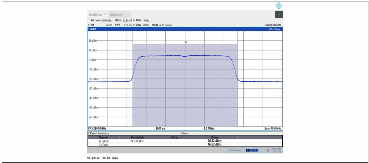
11AX20MIMO_Ant2_5280
