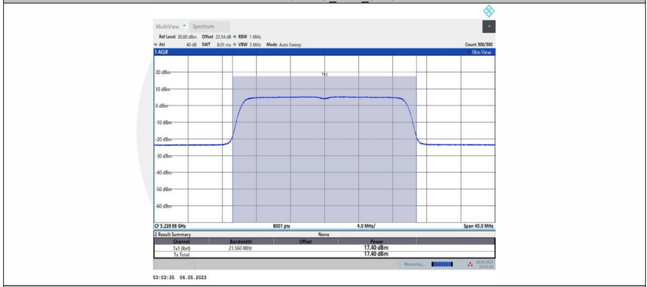
11AX20MIMO_Ant2_5240
