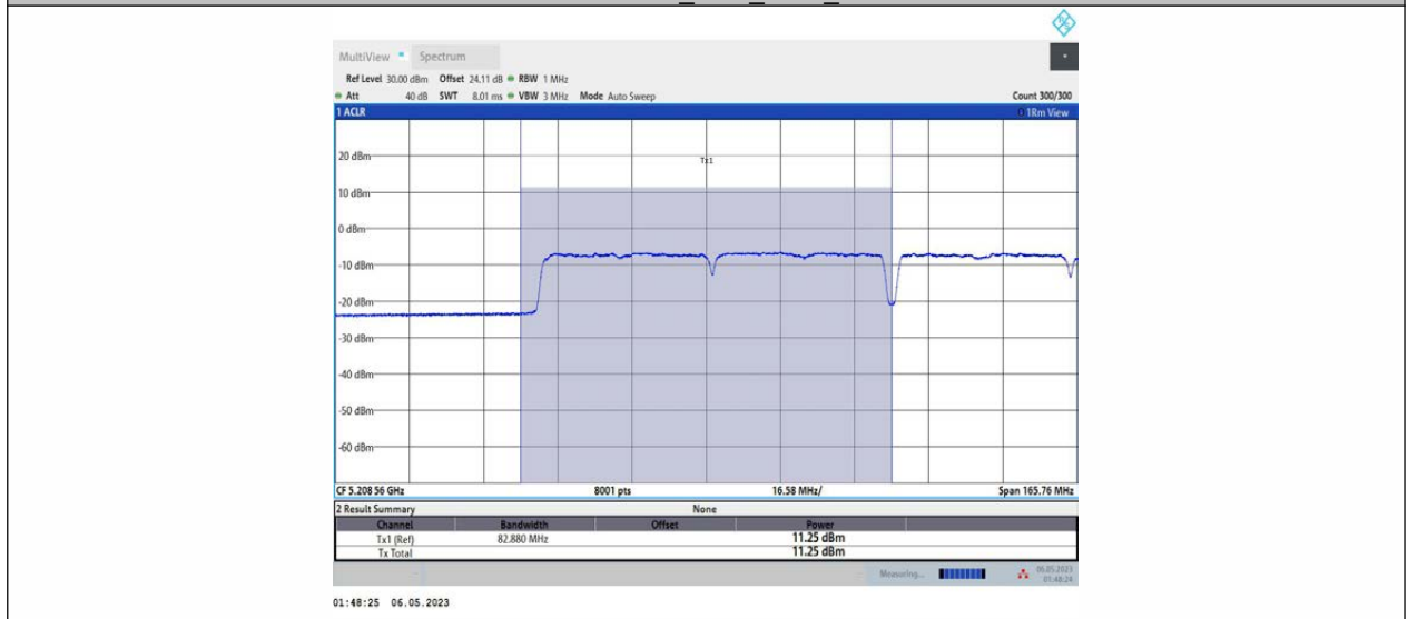
11AC160MIMO_Ant2_5250_UNII-1
