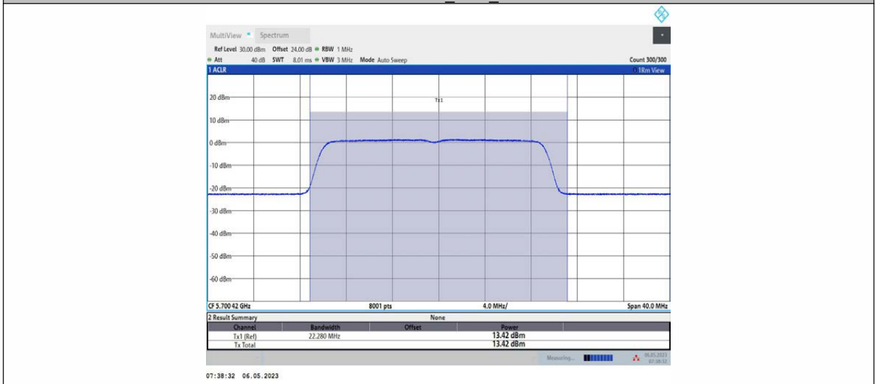
11AX20MIMO_Ant1_5745
