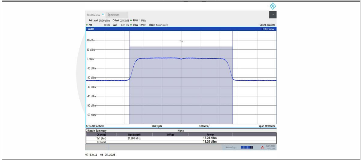
11AX20MIMO_Ant2_5260
