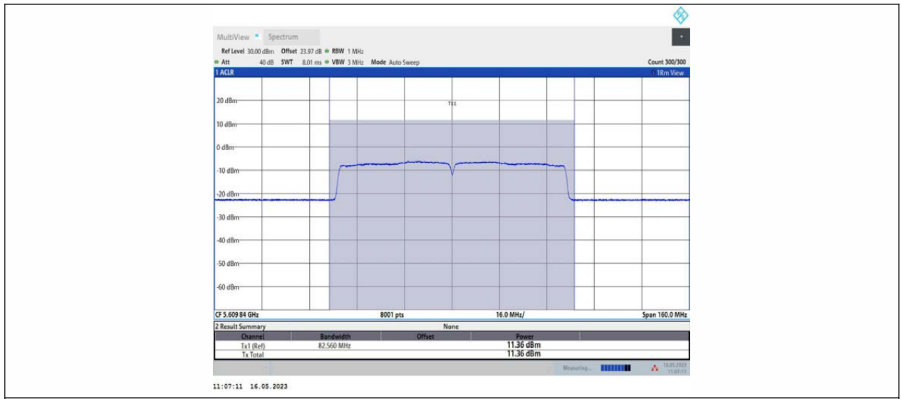
11AC80MIMO_Ant1_5775
