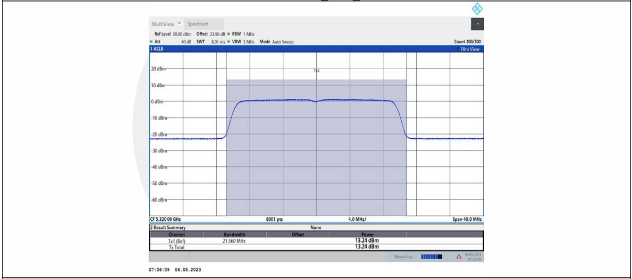
11AX20MIMO_Ant2_5320
