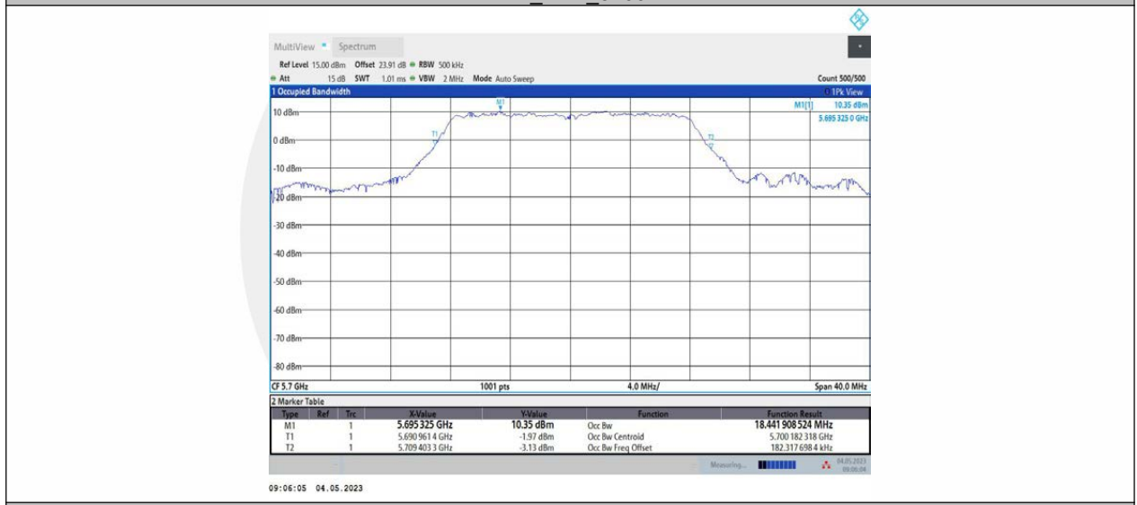
11A_Ant2_5700
