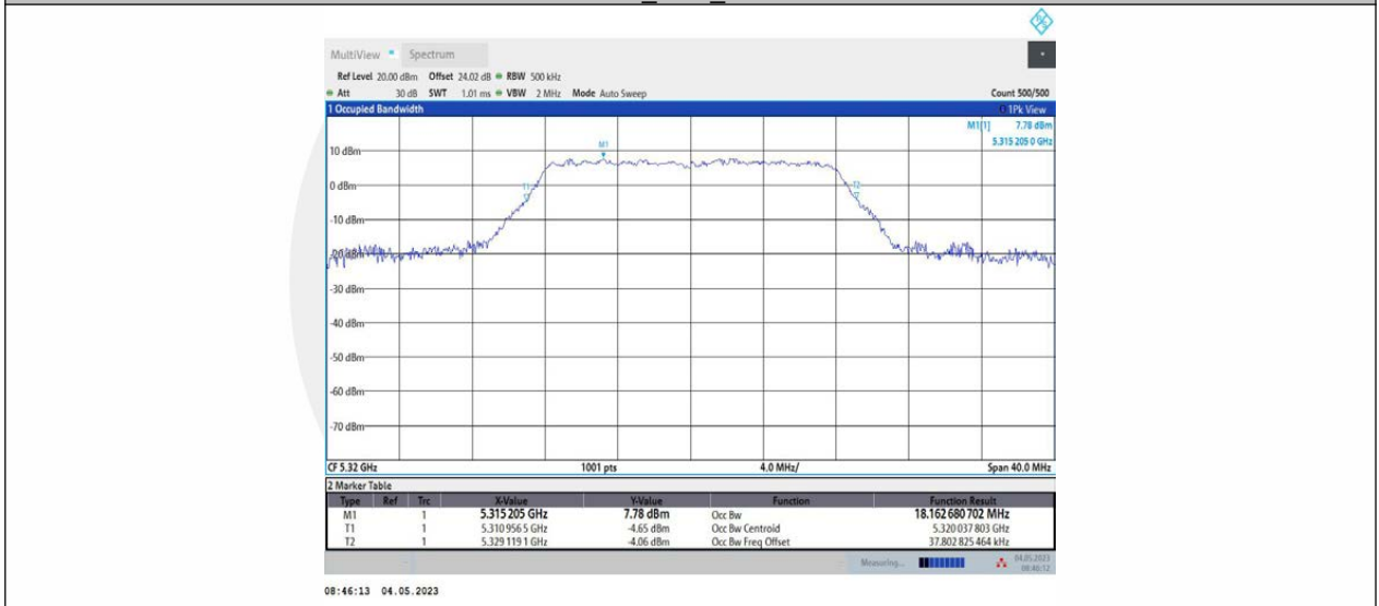
11A_Ant2_5320
