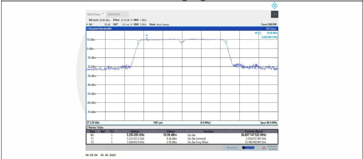
11N40MIMO_Ant2_5550
