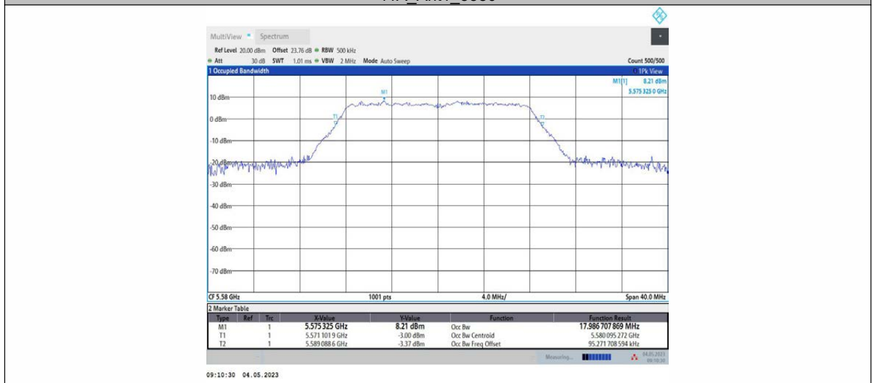
11A_Ant2_5580
