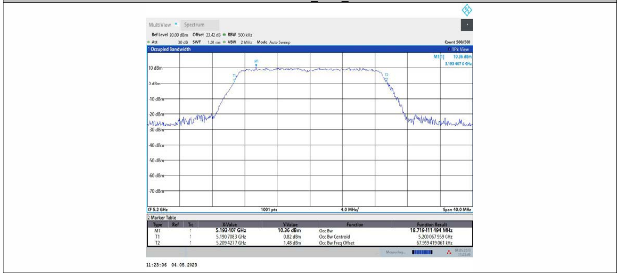
11N20MIMO_Ant2_5200
