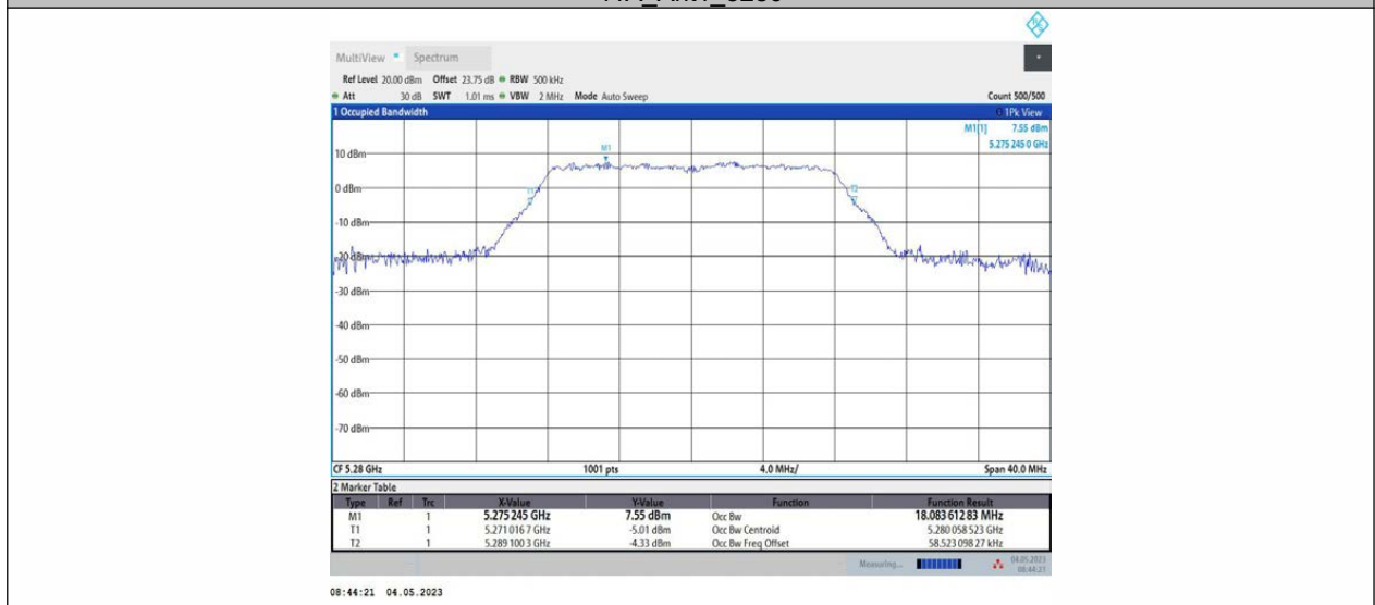
11A_Ant2_5280
