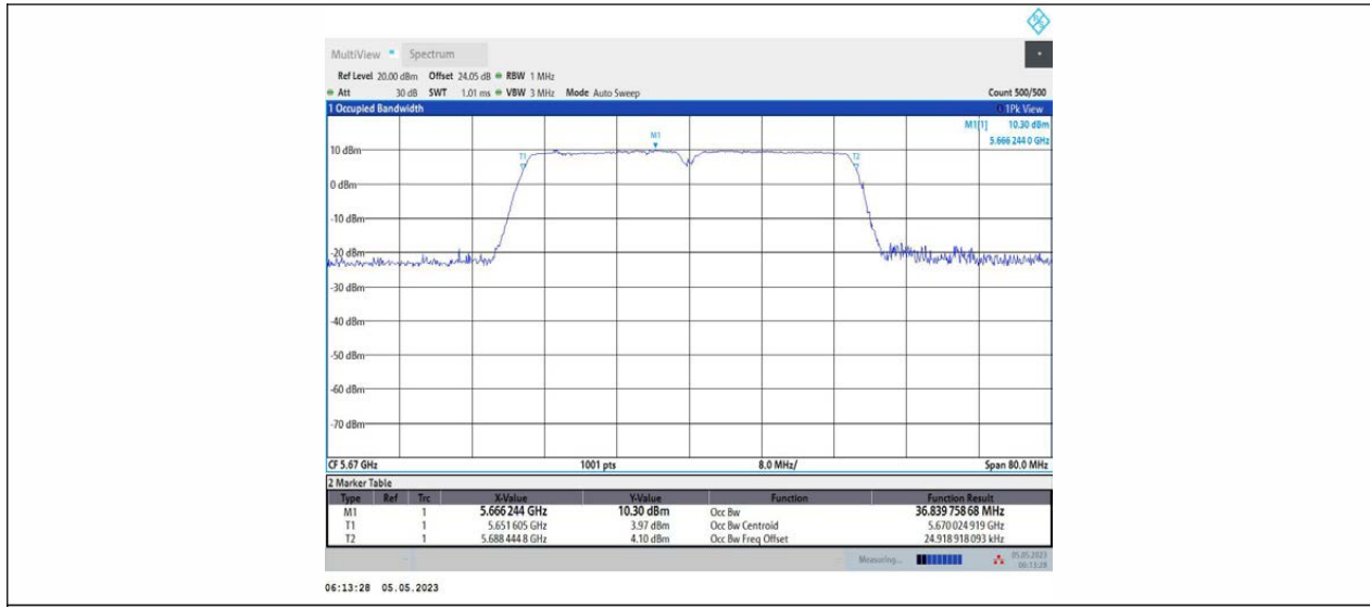
11N40MIMO_Ant2_5670
