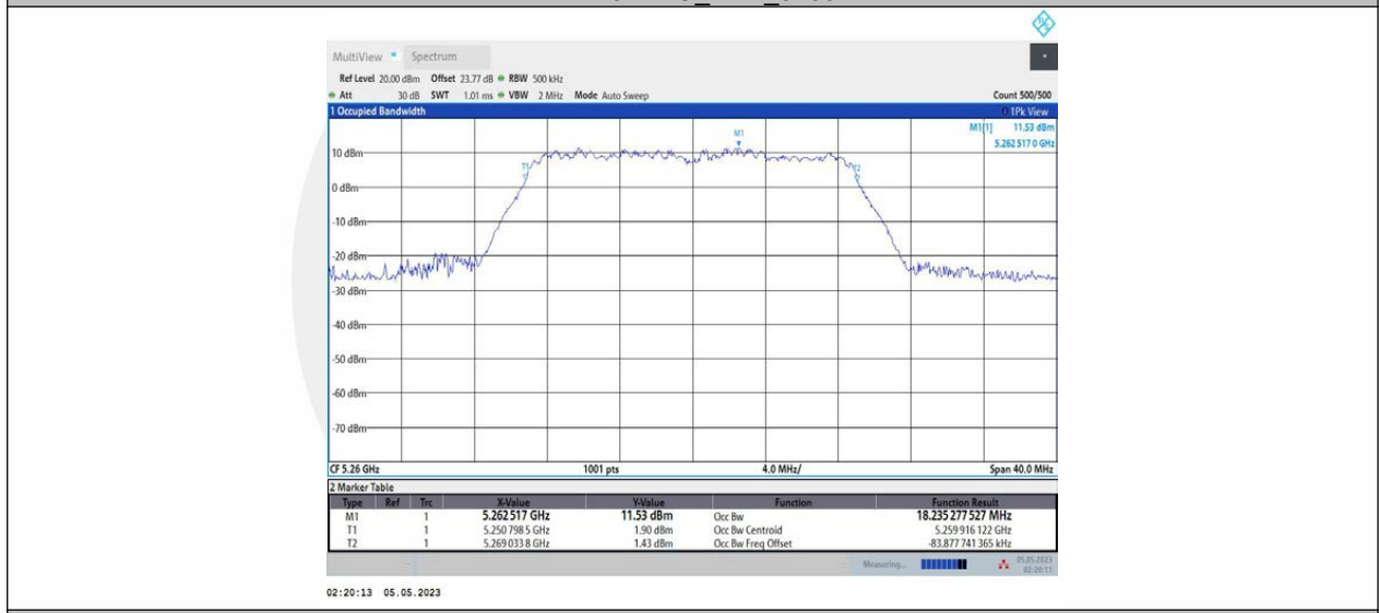
11N20MIMO_Ant1_5280
