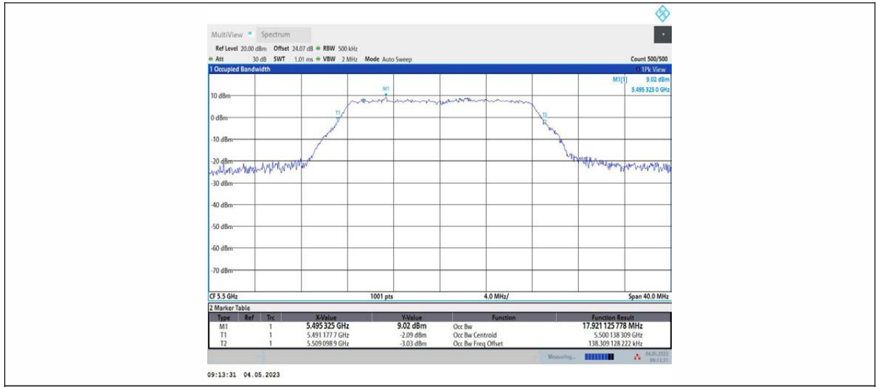
11A_Ant2_5500
