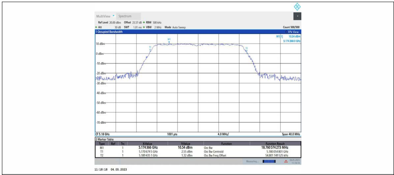
11N20MIMO_Ant2_5180
