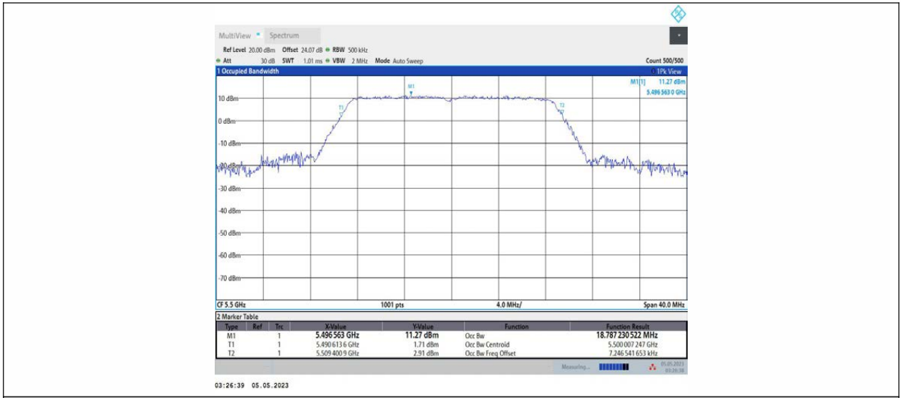
11N20MIMO_Ant2_5500
