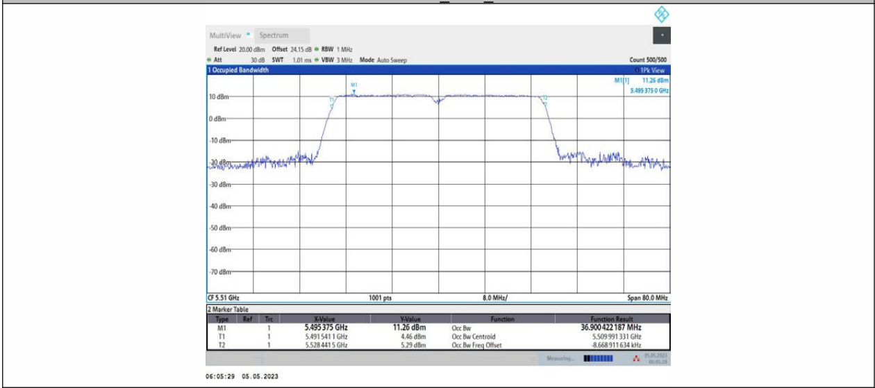
11N40MIMO_Ant2_5510
