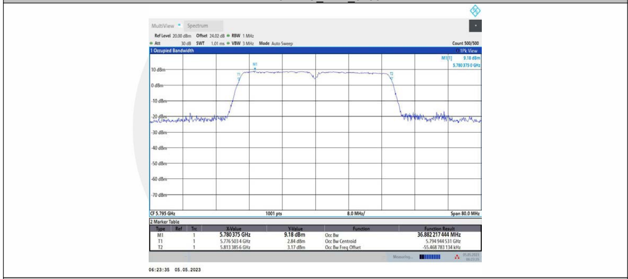
11N40MIMO_Ant2_5795
