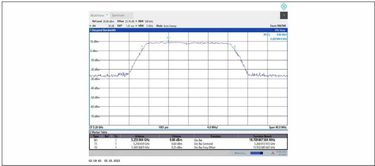
11N20MIMO_Ant2_5260
