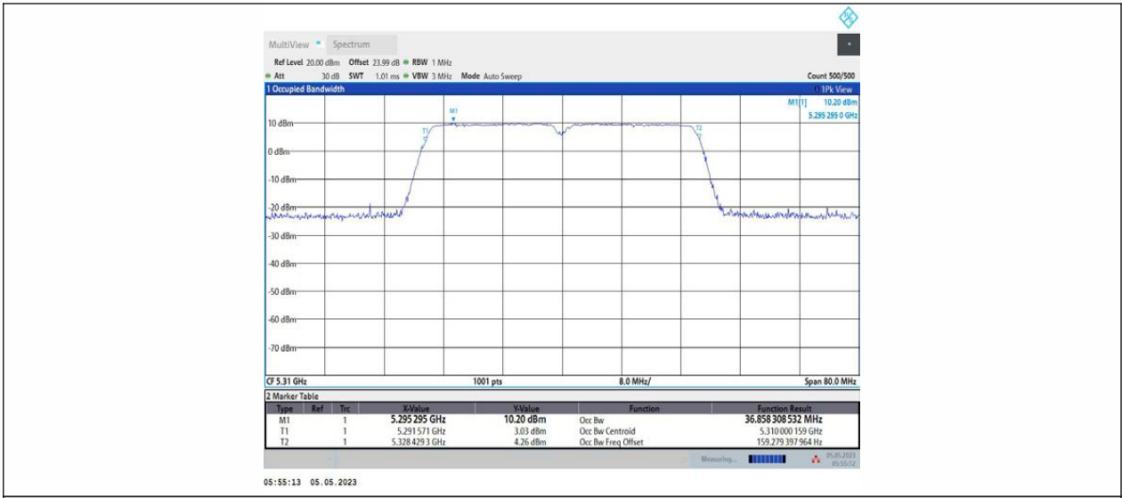
11N40MIMO_Ant2_5310
