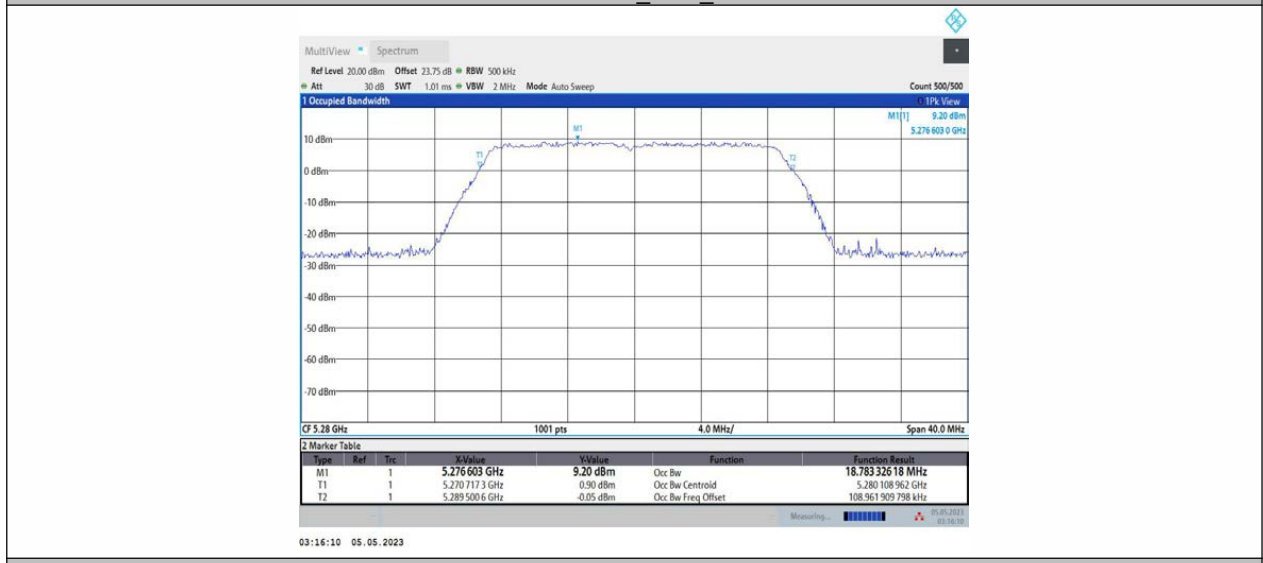
11N20MIMO_Ant2_5280
