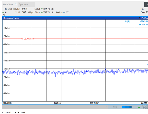
Band25-20MHz-QPSK-26140-1RB#0-Range2:0.15~30MHz
