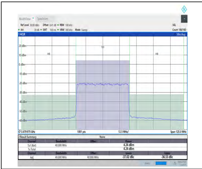
NTNV_N48_PC3_30_40_H_TID16_#1_+40_40
