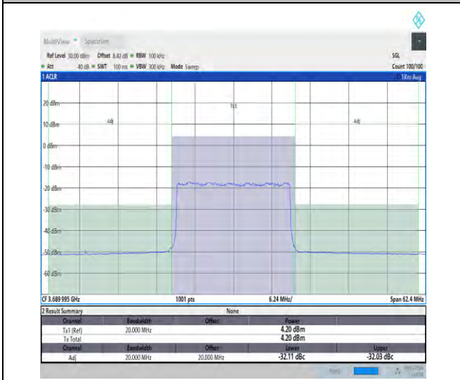
NTVN_N48_PC3_30_20_H_TID16_#1_-20_20
