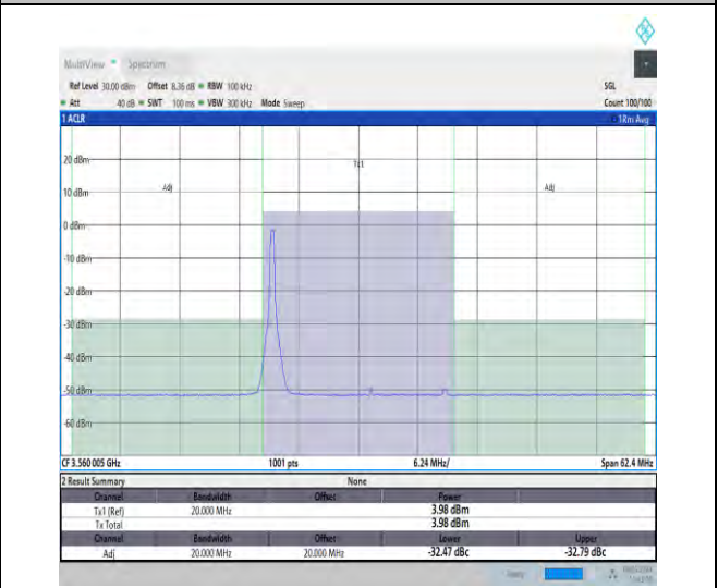
NTVN_N48_PC3_30_20_L_TID17_#1_-20_20
