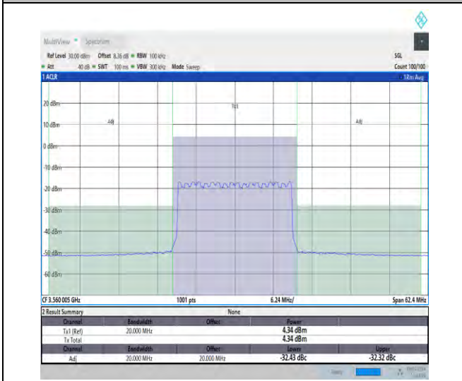
NTVN_N48_PC3_30_20_L_TID16_#1_-20_20
