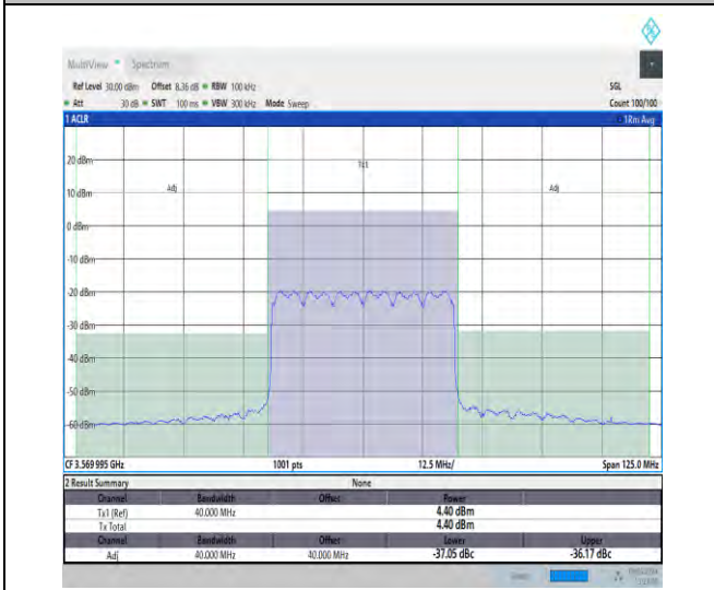
NTVN_N48_PC3_30_40_L_TID16_#1_-40_40
