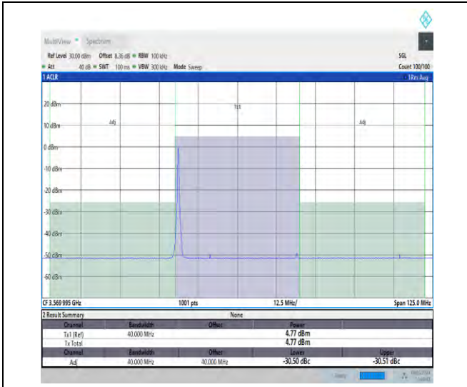
NTVN_N48_PC3_30_40_L_TID17_#1_-40_40
