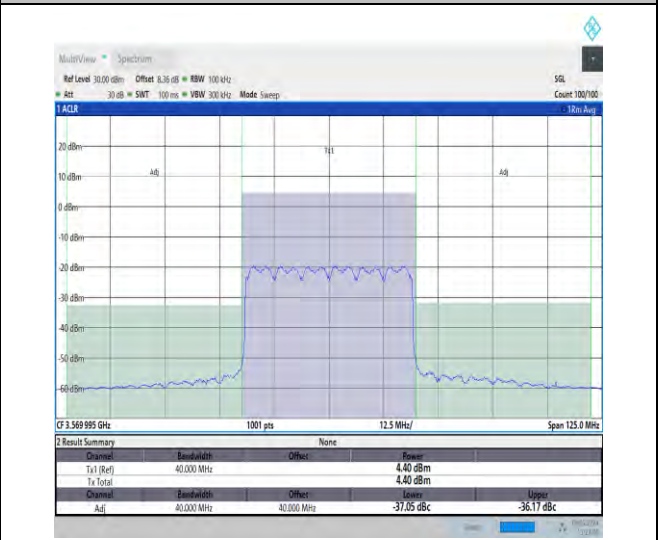
NTVN_N48_PC3_30_40_L_TID16_#1_+40_40
