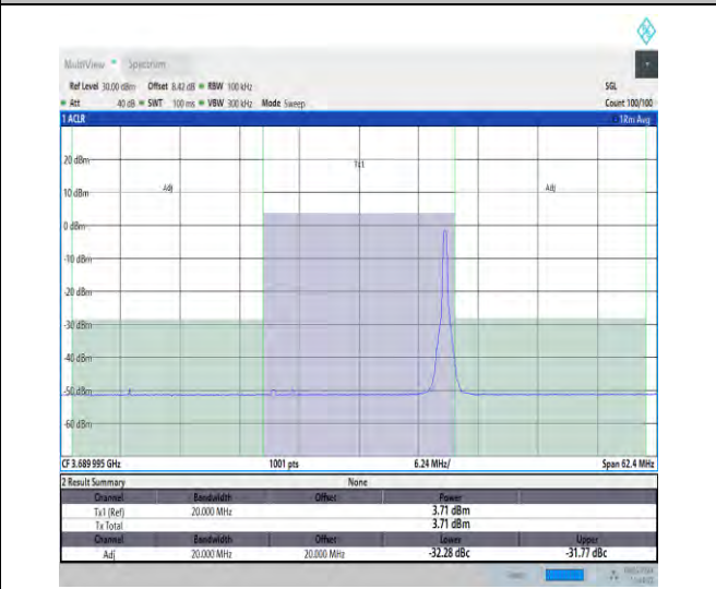
NTVN_N48_PC3_30_20_H_TID18_#1_-20_20
