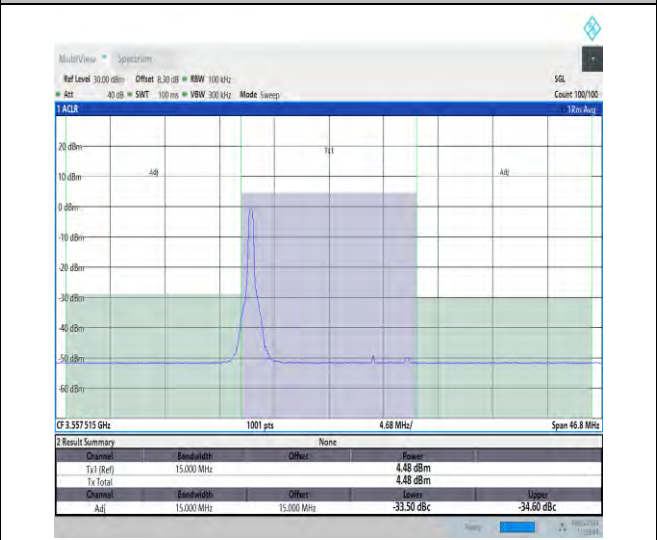
NTVN_N48_PC3_30_15_L_TID17_#1_-15_15
