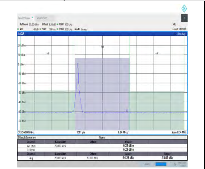
NTVN_N48_PC3_30_20_L_TID2_#1_-20_20
