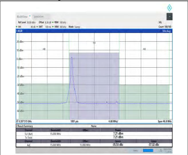
NTVN_N48_PC3_30_15_L_TID2_#1_-15_15
