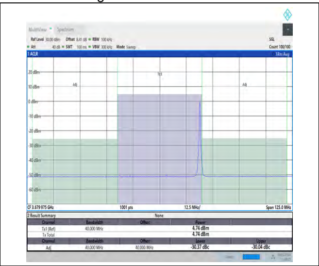
NTNV_N48_PC3_30_40_H_TID18_#1_-40_40
