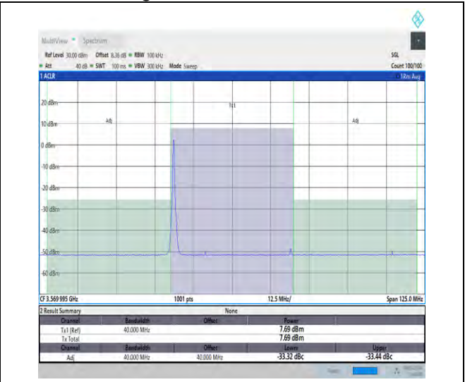
NTVN_N48_PC3_30_40_L_TID2_#1_-40_40
