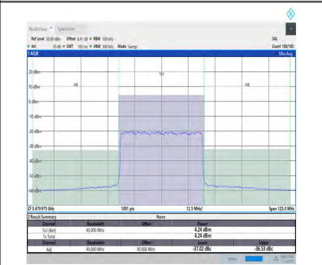
NTVN_N48_PC3_30_40_H_TID16_#1_-40_40
